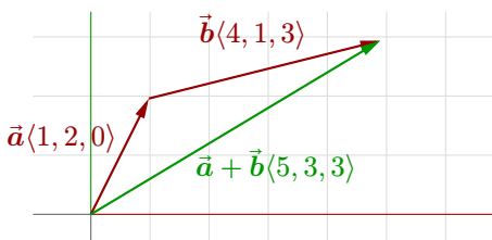
图 8 向量加法
