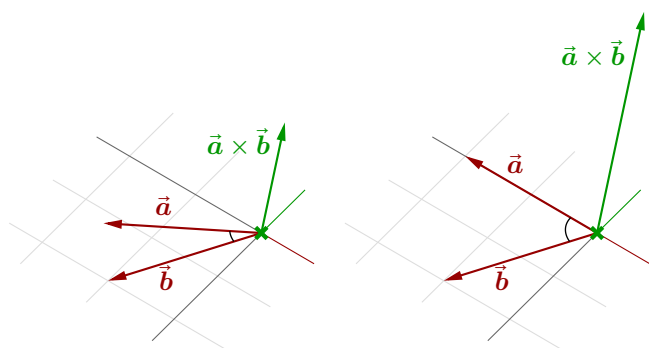
图 15 两个向量夹角的正弦和叉积的模之间的关系
