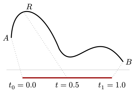
图 26 归一化曲线区间到 0 到 1
