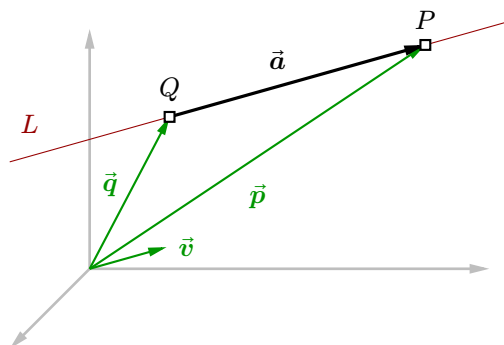
图 16 直线的矢量方程
