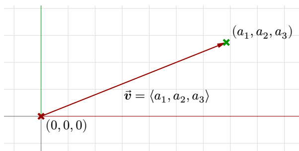
图 3 位置向量, 端点坐标等于向量坐标
