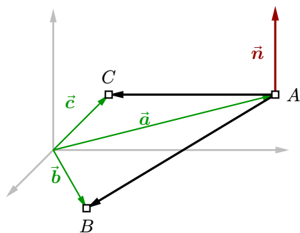
图 18 向量和平面
