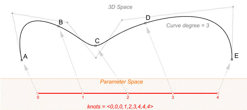
图 36 控制点、节点列表长度和阶数的关系
