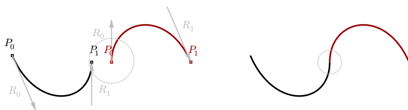
图 32 两个 Hermite 曲线段共用一个点和一个切线
