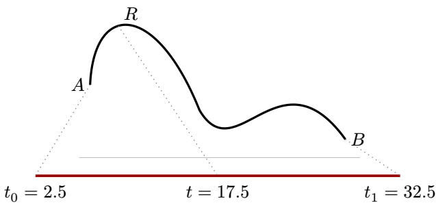
图 25 曲线区间介于任意两数之间
