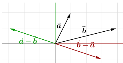
图 10 向量减法
