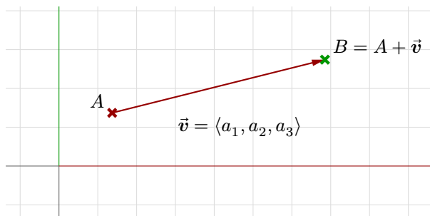
图 2 向量、向量起始点、向量结束位置所在点之间的关系
