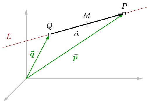
图 17 找到两点之间的中点
