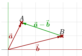
图 11 使用向量减法找到两点之间的向量
