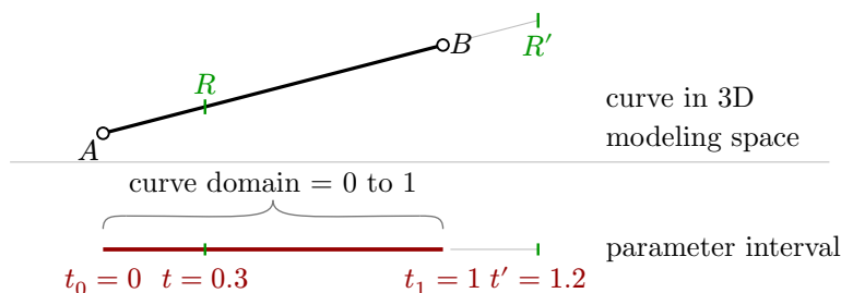
图 23 三维空间和参数区间中的线段的参数曲线
