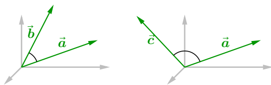
图 12 当两个向量同方向时，结果是正点积（左），当两个向量不同方向时，结果是负点积（右）
