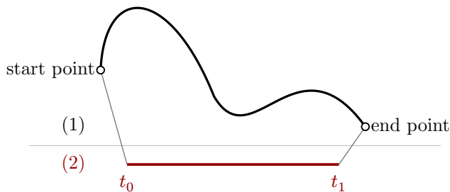
图 24 三维空间 (1) 和参数区间 (2) 中的曲线
