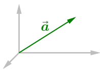
图 5 向量长度
