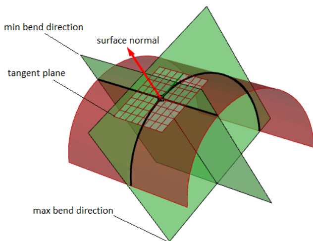
图 58 法向曲率
