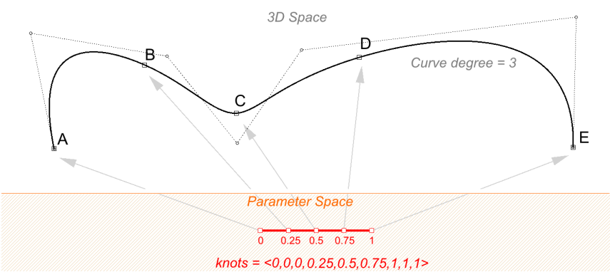
图 37 缩放节点列表后的曲线
