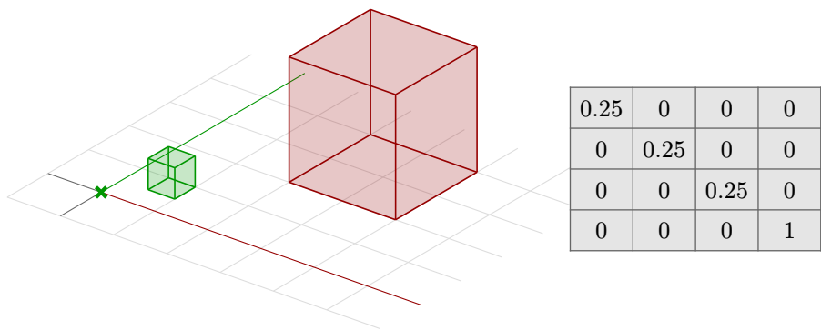
图 21 缩放几何
