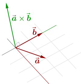
图 14 计算两个向量的叉积
