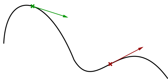
图 29 曲线的切线
