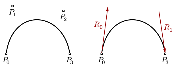
图 30 三次多项式曲线：Bezier 曲线（左）和 Hermite 曲线（右）
