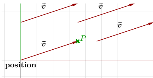
图 4 向量定义方向和长度，点定义位置
