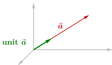
图 6 单位向量等于一个单位长度的向量
