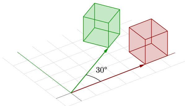
图 20 旋转几何
