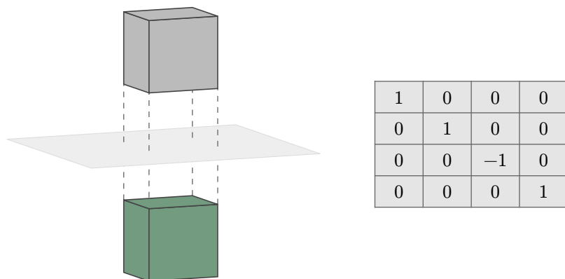
图 22 使用世界坐标 xy 平面镜像变换的矩阵, 面法向被翻转
