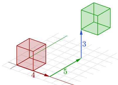
图 19 平移所有方框角点
