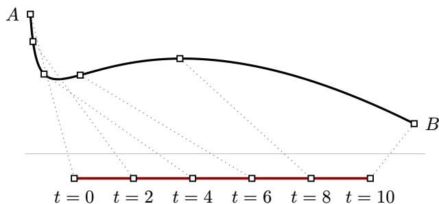
图 28 相等的参数间隔通常不会转换为曲线上的相等距离
