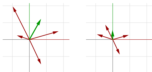
图 9 对不同长度向量求和（左）对相同长度向量求和（右）来获得平均方向
