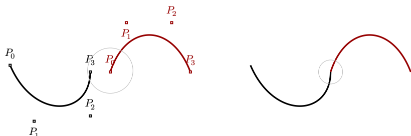
图 31 两个 Bezier 曲线段共用端点
