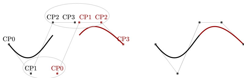
图 33 两个 3 次 NURBS 曲线段共享三个控制点。
