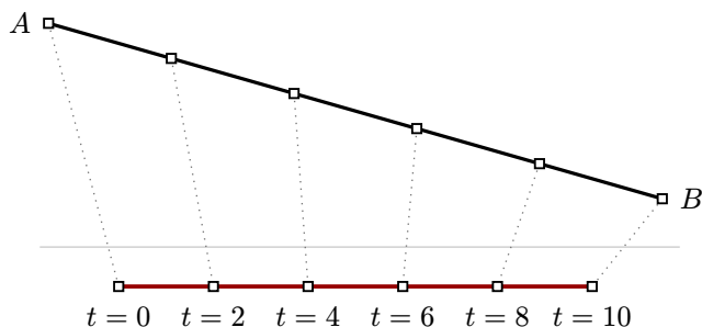
图 27 一阶直线相等的参数间隔计算为相等的曲线长度
