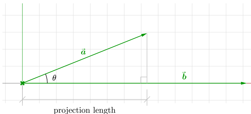
图 13 一个向量的投影长度是一个向量和另一个向量的单位向量的点积
