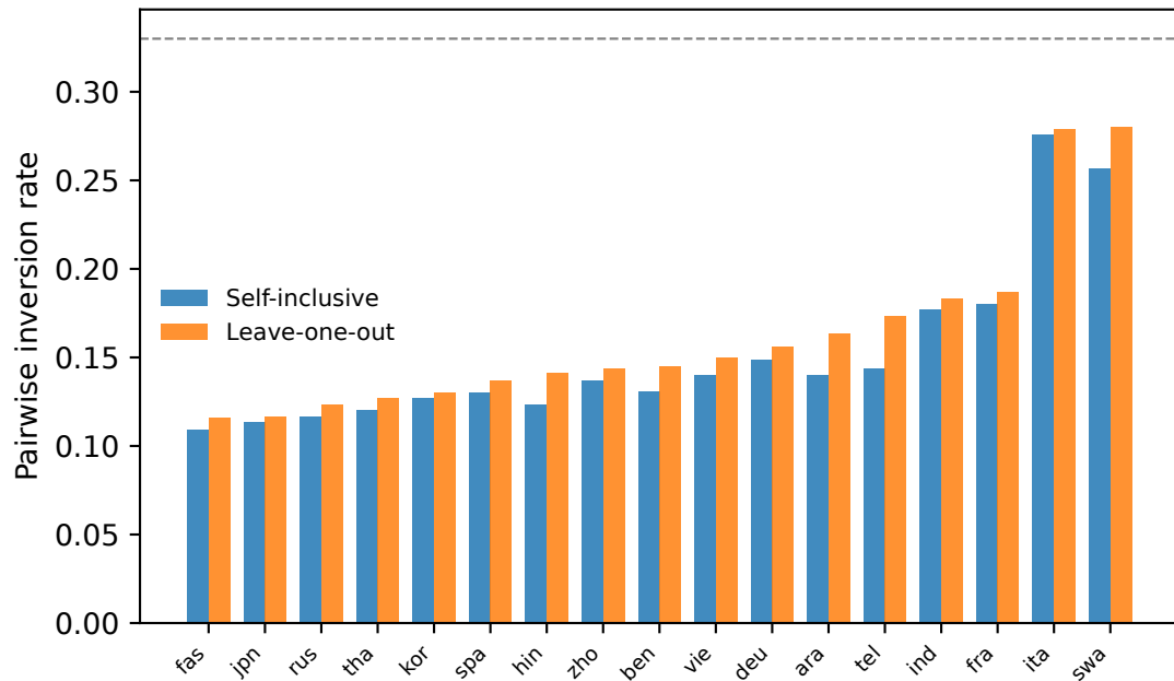
Lang-macro 18lang
