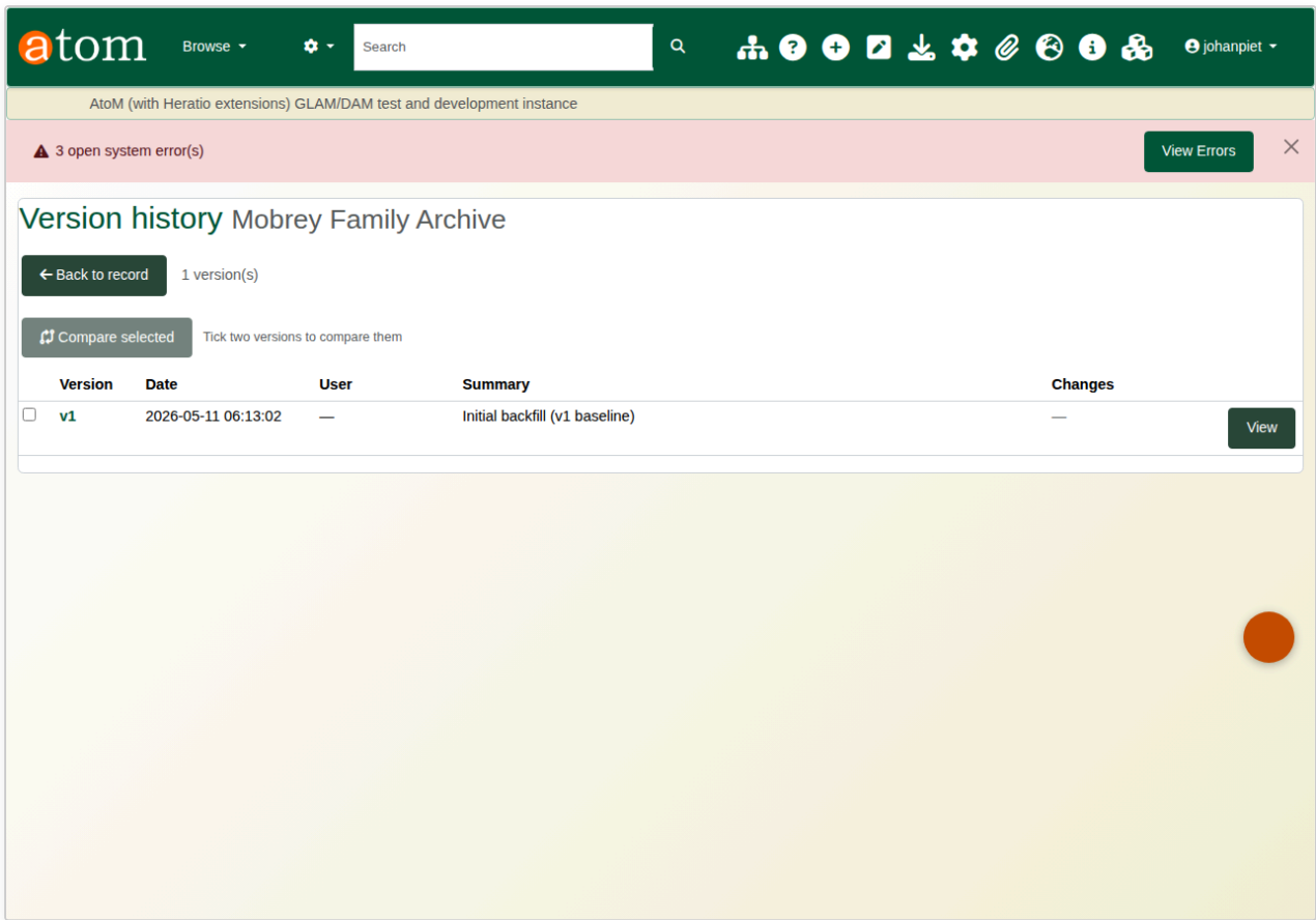
S8-version-restore.png
