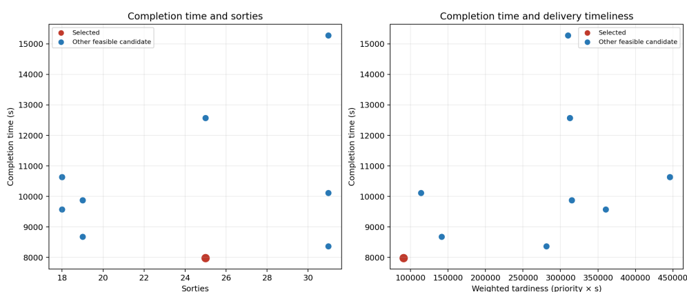
图 8 问题二候选方案在全部完工时间、出动架次与加权迟到量之间的多目标权衡散点图
