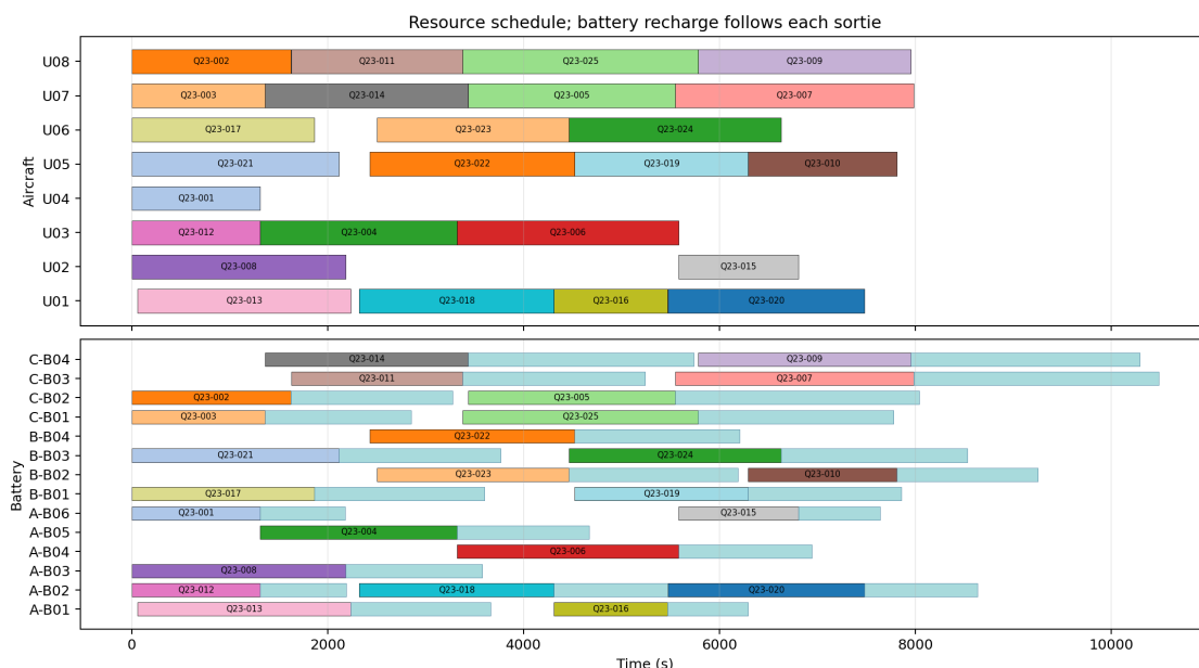
图 6 问题二 8 架实体无人机与 14 组共享电池协同调度与充放电周转甘特图
