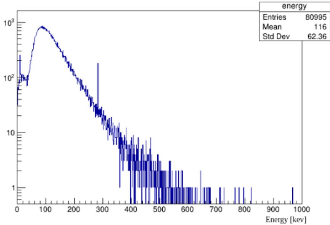
Gambar 2.5 Spektrum energi dari Cesium-137 [59]
