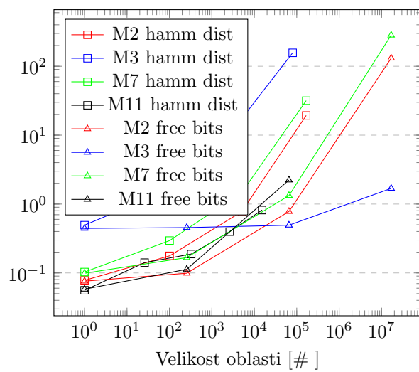
Závislost délky výpočtu na velikosti vstupní oblasti
