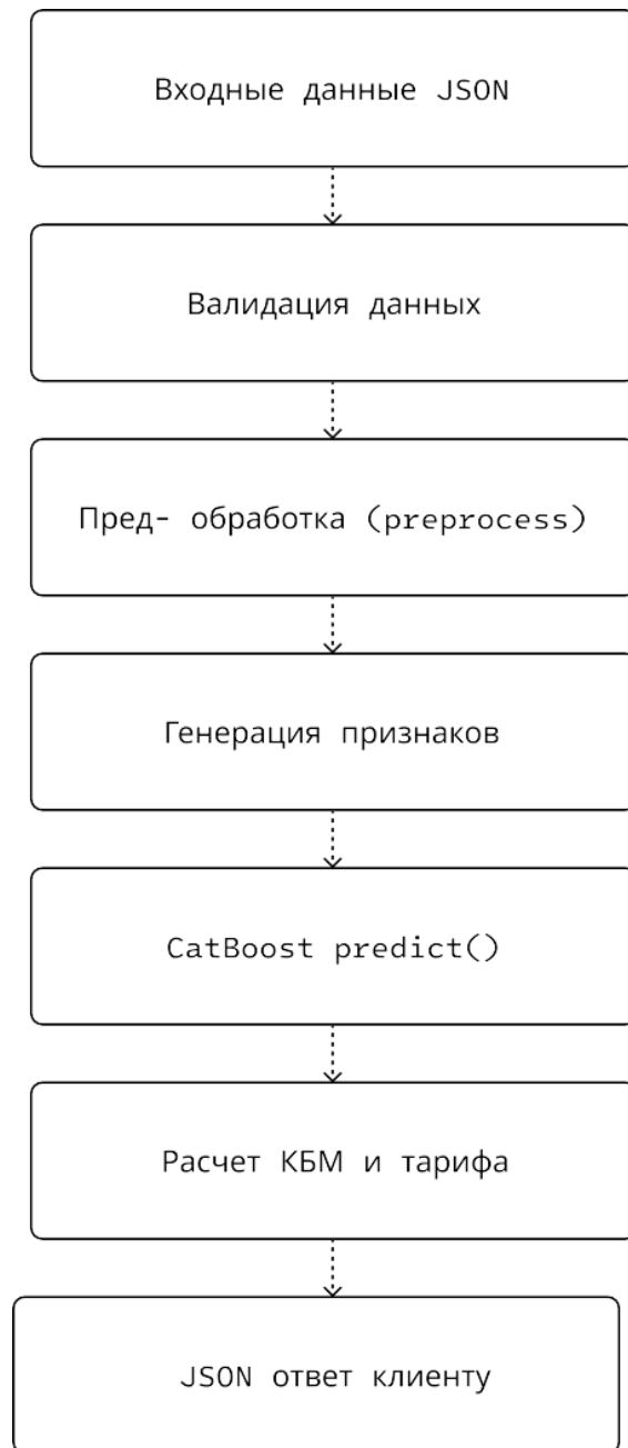
Рис. 2.4 – Блок-схема серверного конвейера обработки запросов
