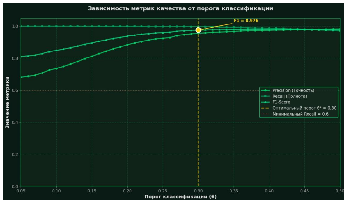
Рис. Приложение .7 — Зависимость метрик качества (Precision, Recall, F1-score) от порога классификации \theta
