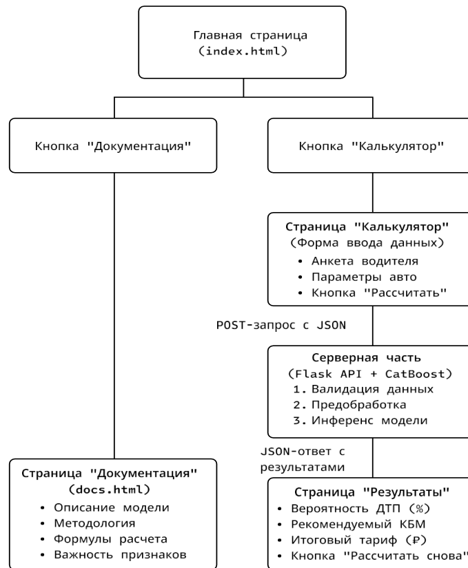
Рис. 2.2 – Структурная схема веб-приложения с указанием навигационных связей и потоков данных
