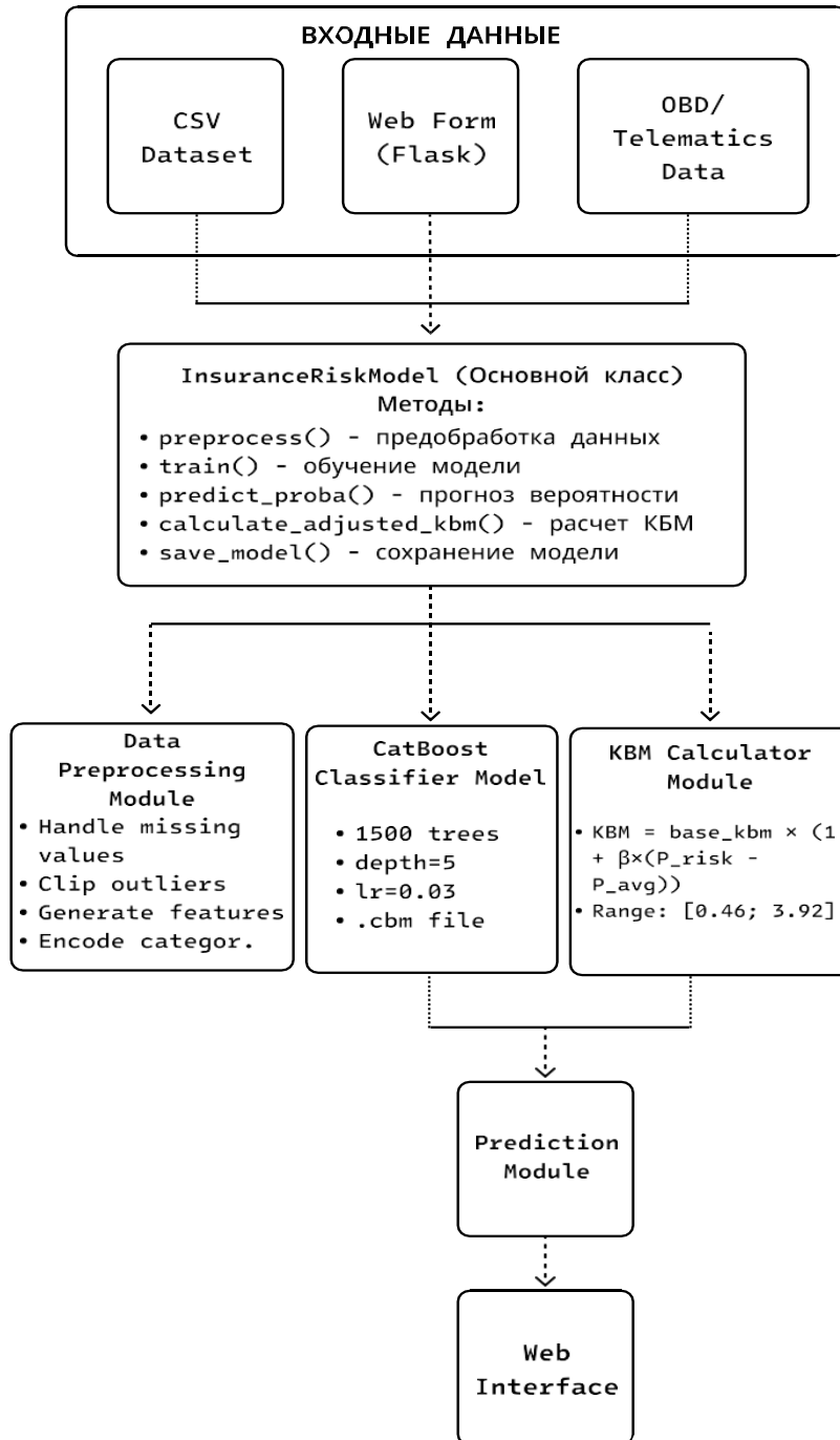
Рис. 2.1 – Архитектурная схема системы прогнозирования страховых рисков
