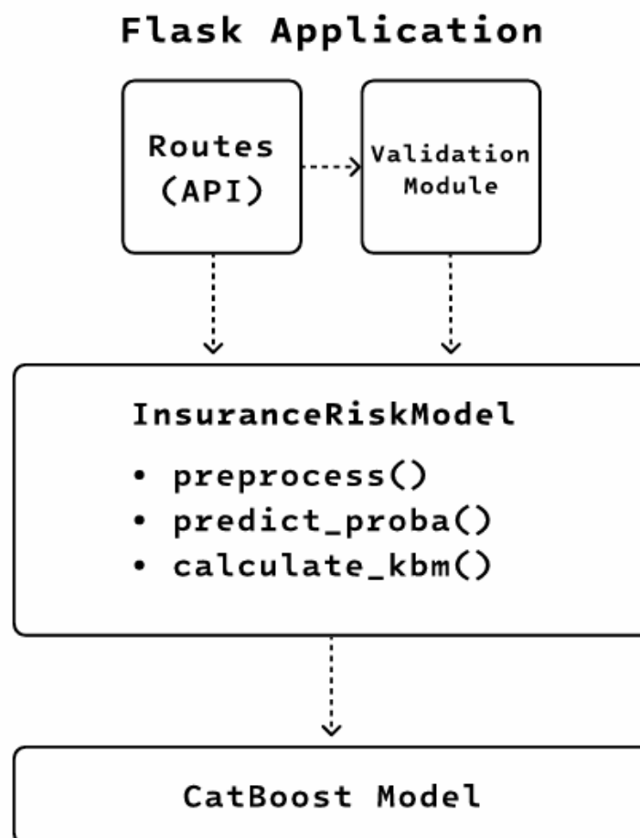
Рис. 2.3 – Схема архитектуры серверной части веб-приложения
