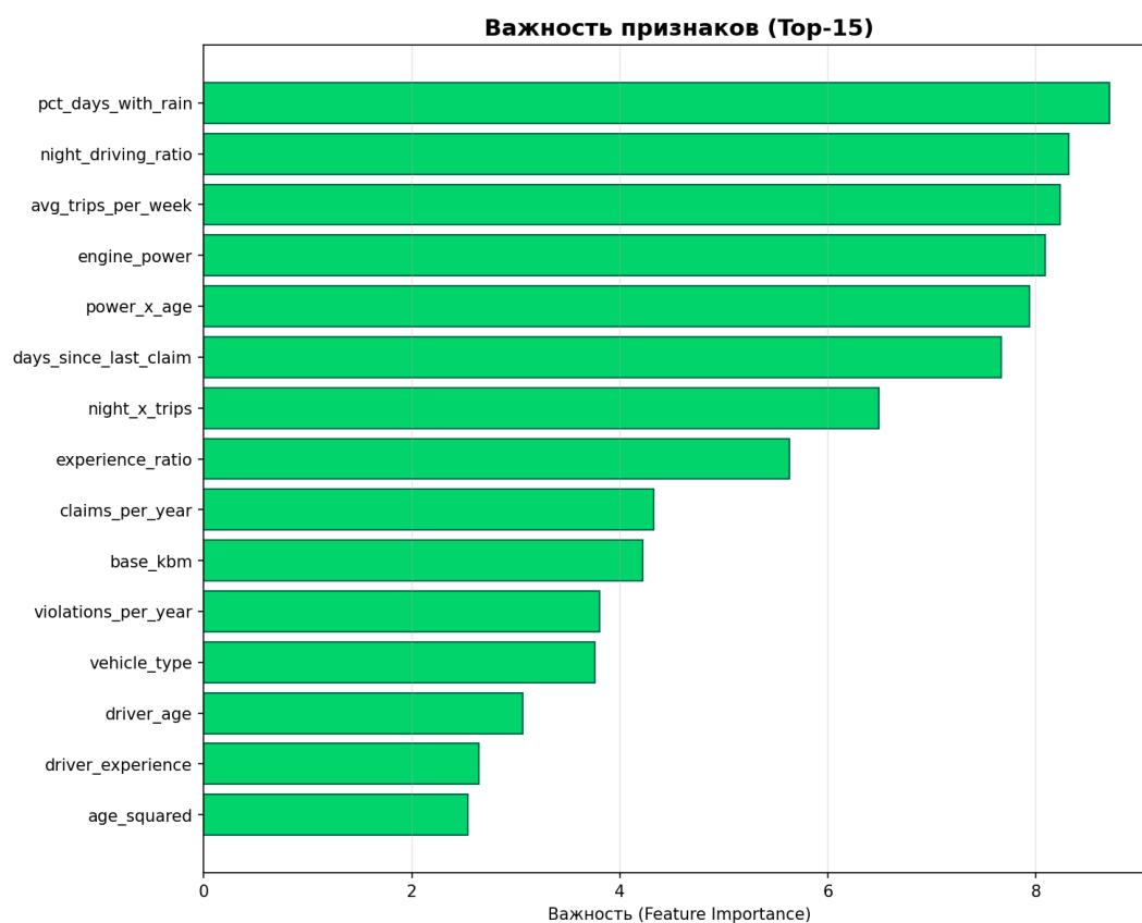
Рис. Приложение .8 — Ранжирование признаков по степени влияния на прогноз
