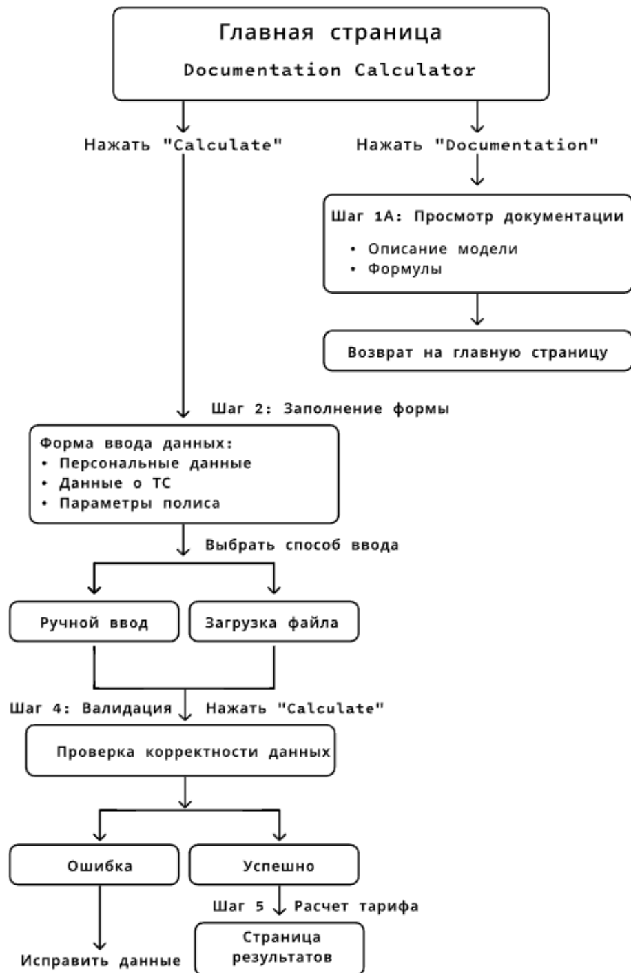
Рис. 2.6 – Диаграмма пользовательского сценария
