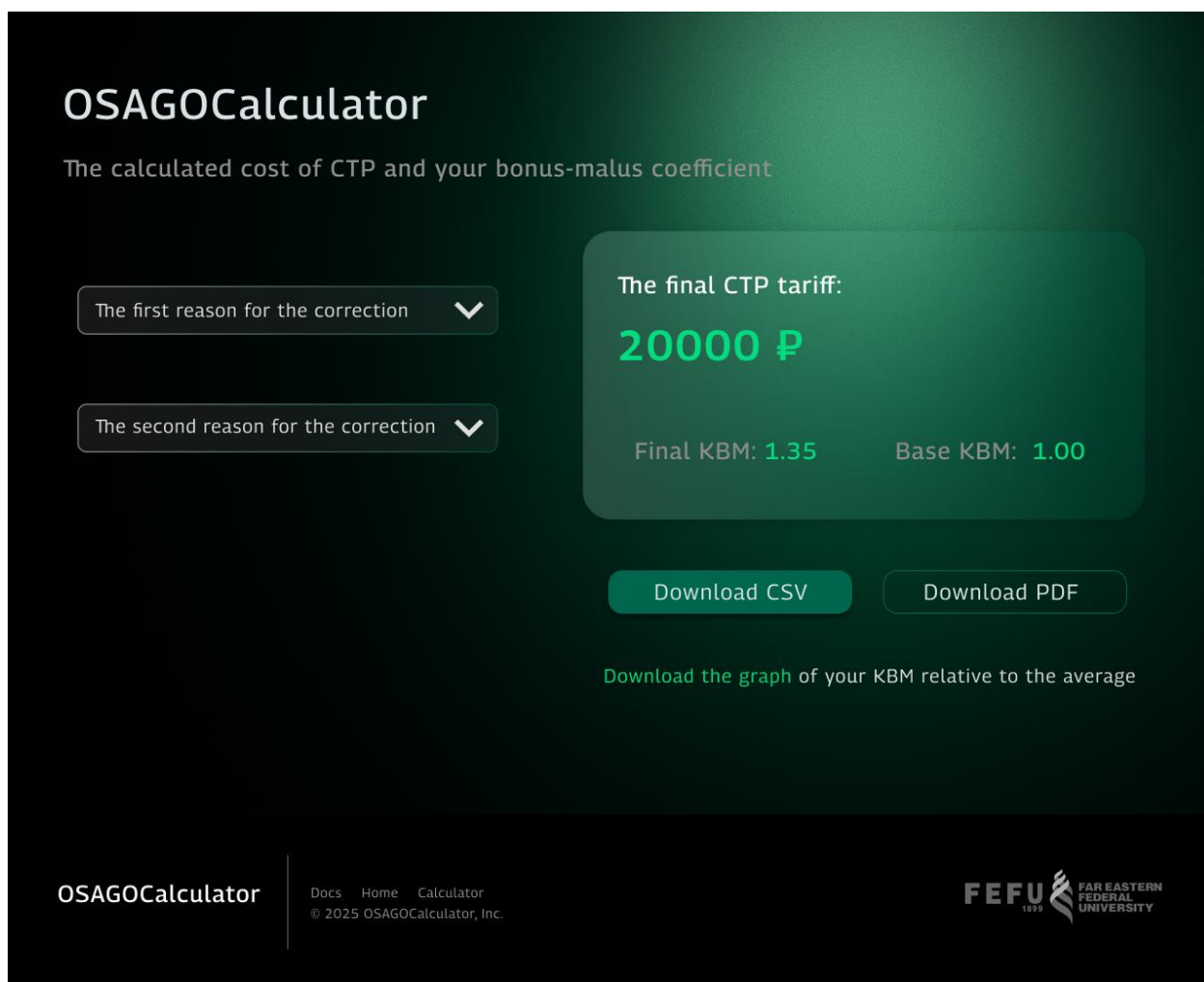
Рис. Приложение .16 – Отображение финального тарифа и коэффициентов КБМ
