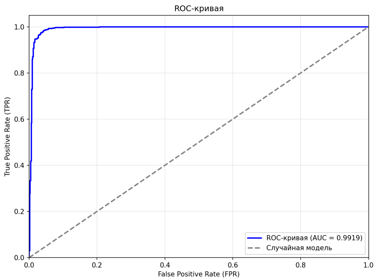
Рис. Приложение .10 – ROC-кривая классификатора
