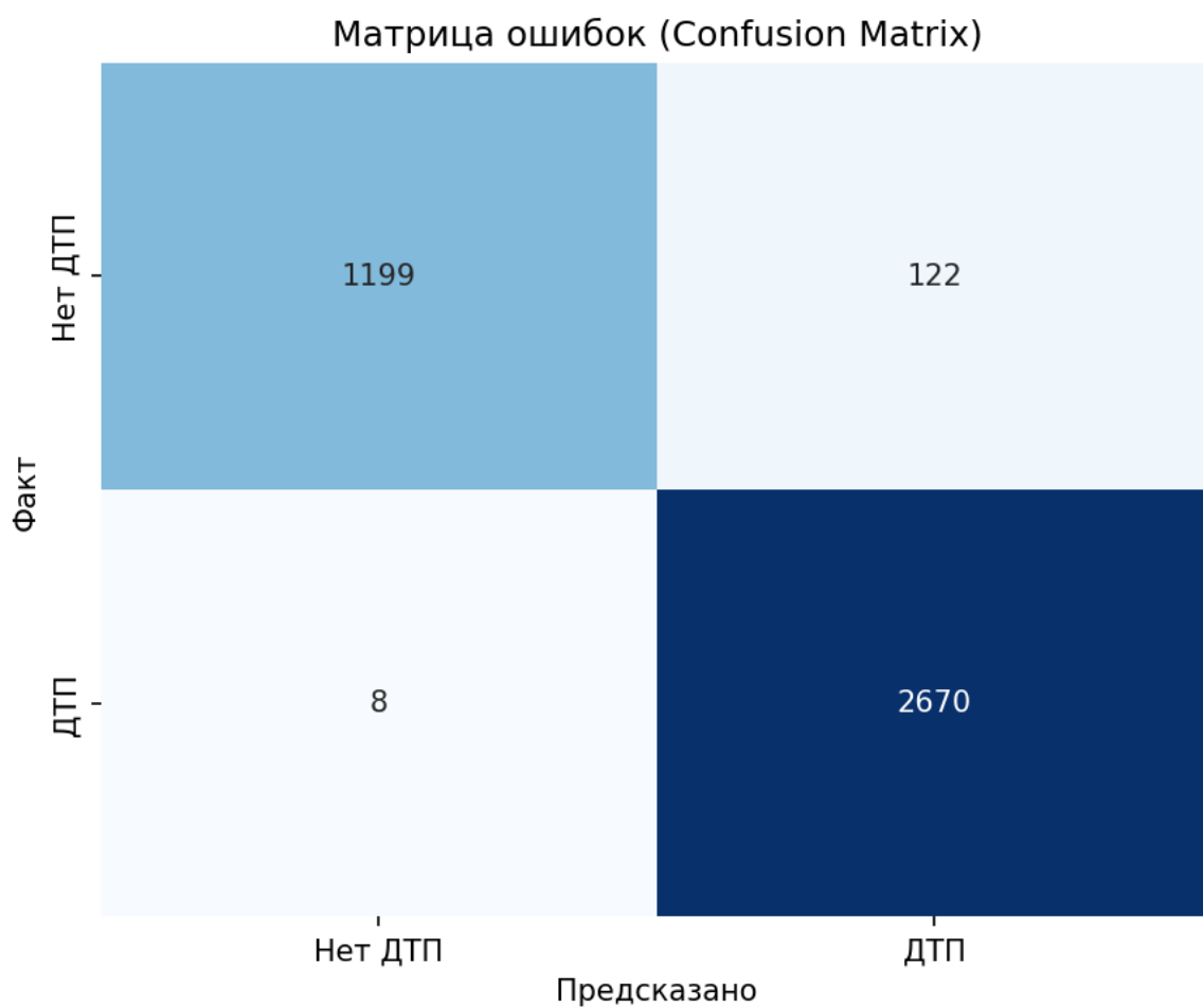
Рис. Приложение .9 – Распределение прогнозов модели
