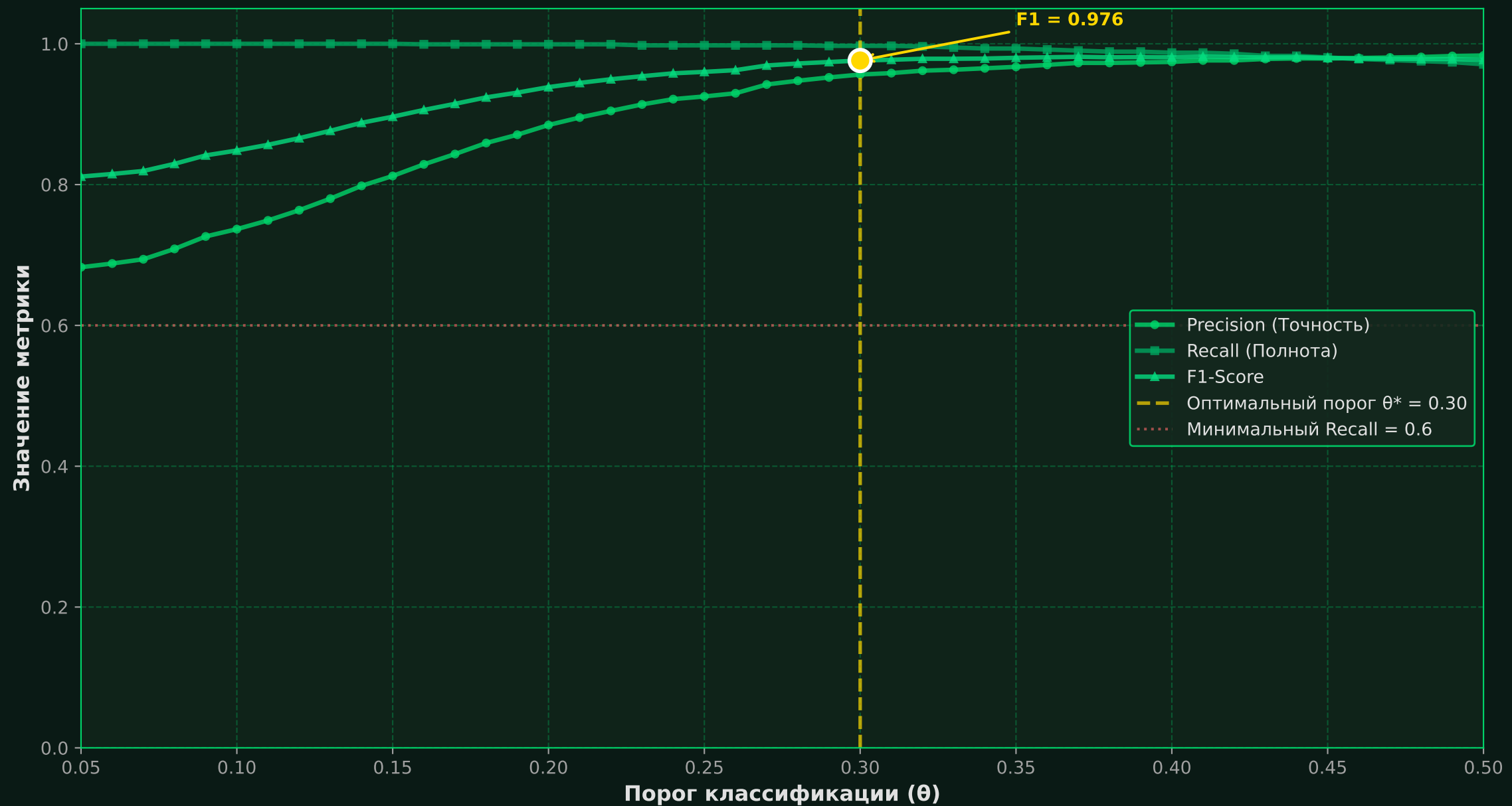
Зависимость метрик качества от порога классификации
