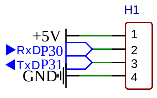
下载口
