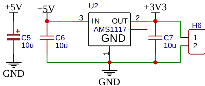
3.3V线性稳压电源
