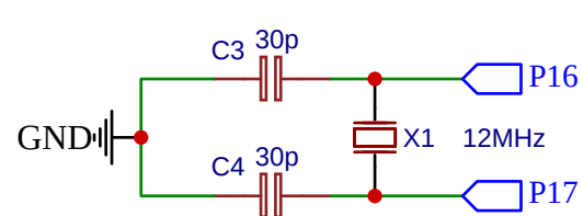
晶振电路
