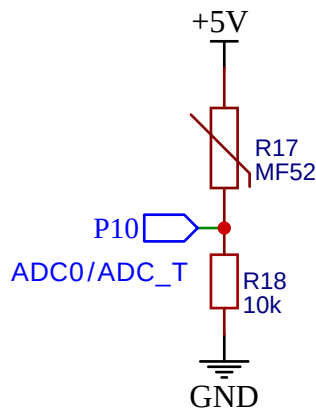
NTC测温
