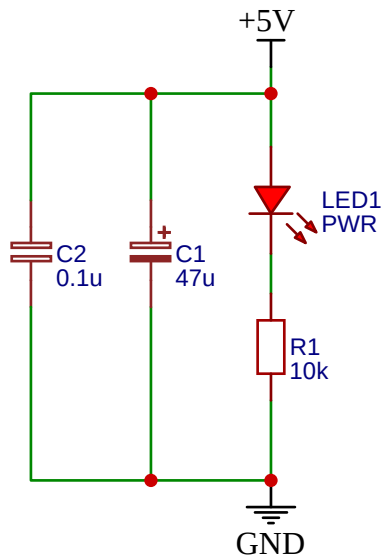
电源滤波与指示灯
