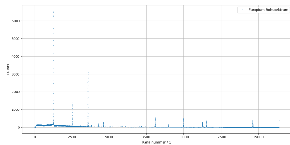
(b) HPGe-Halbleiterdetektor
