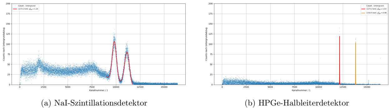
Abbildung 5.1: Gemessenes Energie-Spektrum der ^{60}\text{Co} -Quelle an beiden Detektoren
