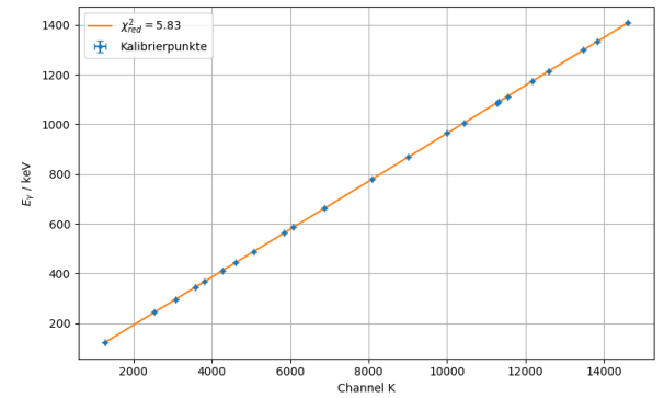
(b) HPGe-Halbleiterdetektor
