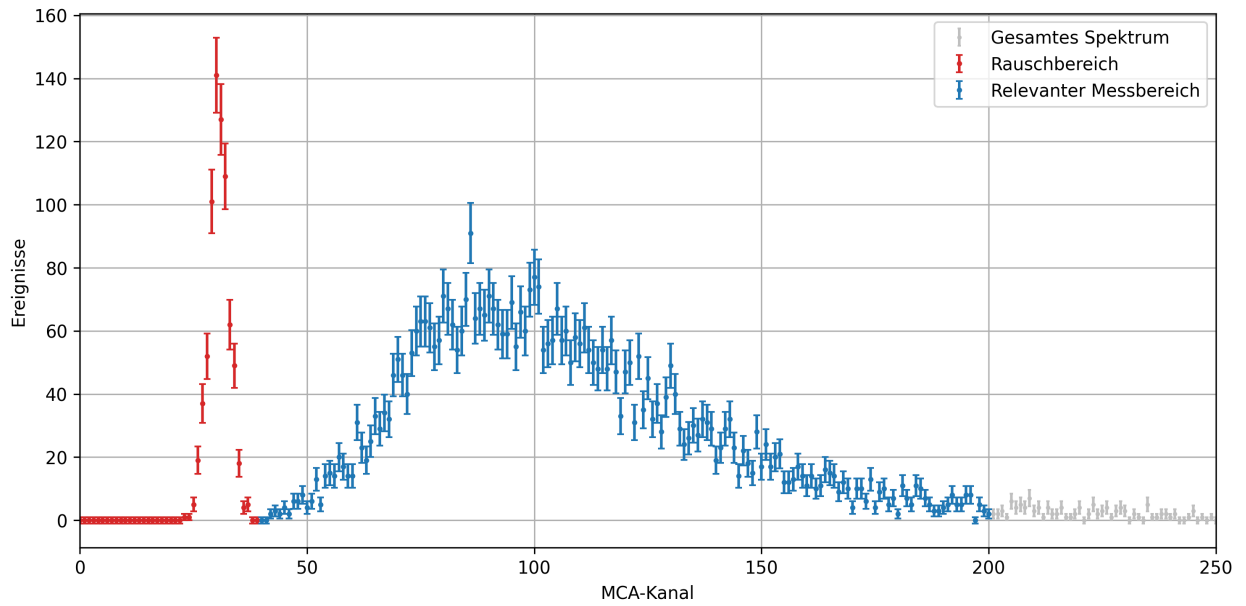
Abbildung 3.6: Rohdaten der Langzeitmessung des Pulshöhenspektrums
