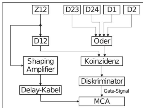
Abbildung 3.4: chaltung zur Aufnahme des PULshöhenspektrums.[2]
