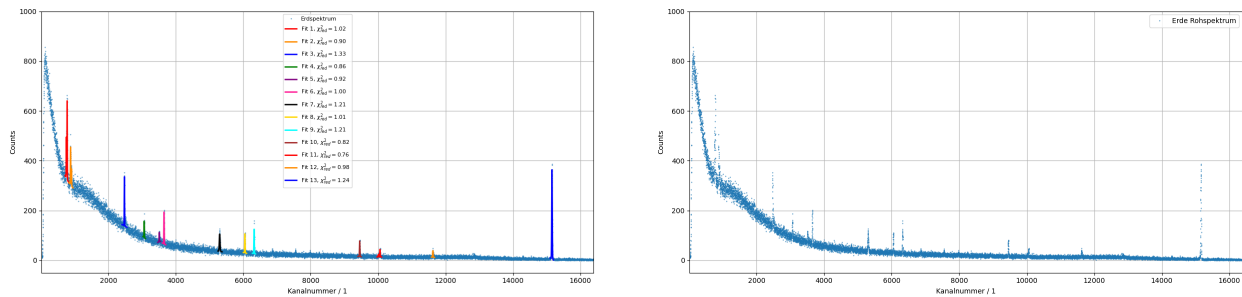
Abbildung 12.5: Am HPGe-Detektor gemessenes Langzeit-Spektrum mit der Bodenprobe.
