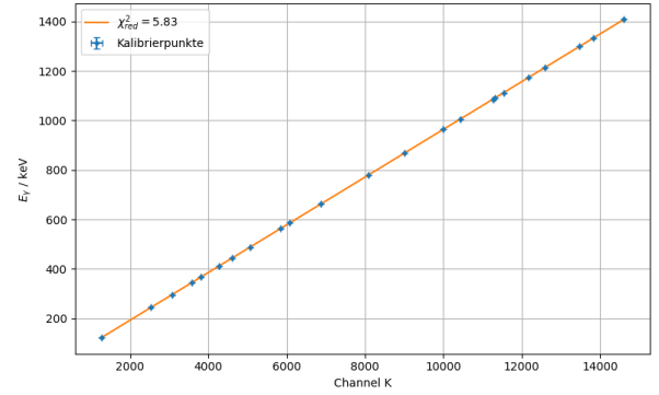
(b) HPGe-Halbleiterdetektor
