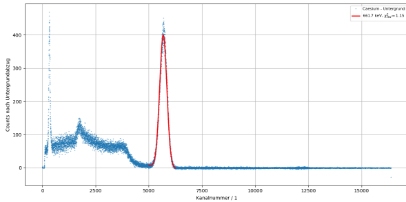
(a) NaI-Szintillationsdetektor
