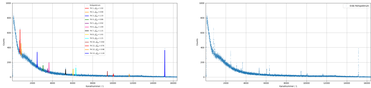
Abbildung 10.6: Am HPGe-Detektor gemessenes Langzeit-Spektrum mit der Bodenprobe.
