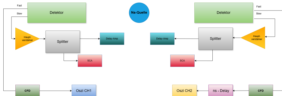
Abbildung 4.6: Schaltplan zur Einstellung der Verzögerung von Start- und Stopp-Signalen im Fast-Kreis.
