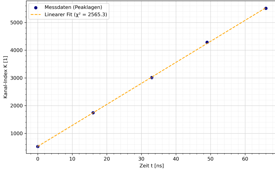
Abbildung 3.12: Zeit-Kanal-Zuordnung von ^{22}\text{Na}
