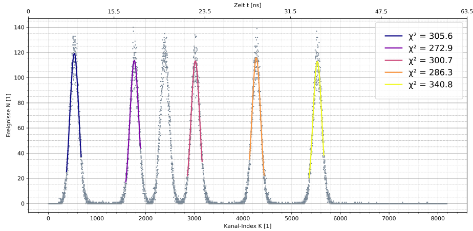
Abbildung 3.11: Messung der Promptkurve mit ^{22}\text{Na} am MCA
