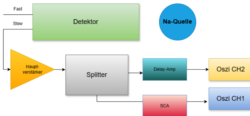
Abbildung 2.4: Schaltplan zur Untersuchung des Hauptverstärkers.
