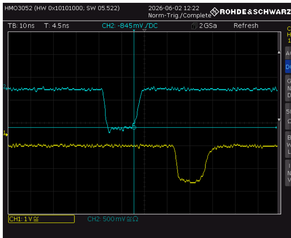
Abbildung 3.8: Oszillogramm des linken Fast-Signals über den CFD (CH 1) im Vergleich zu rechten Fast-Signal über CFD und ns-Delay (CH 2), wobei das ns-Delay auf 31.5ns eingestellt ist. Die Signale sind nun zeitlich so ausgerichtet, dass sie innerhalb des Koinzidenzfensters liegen.
