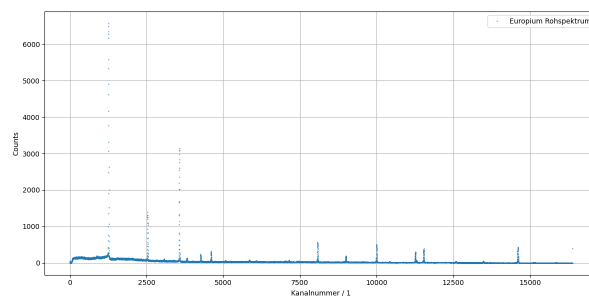
(b) HPGe-Halbleiterdetektor
