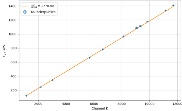
(a) NaI-Szintillationsdetektor
