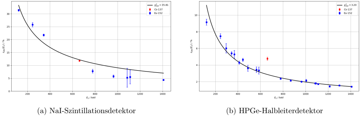
Abbildung 8.1: Effizienz \epsilon(E_\gamma) der Detektoren anhand des ^{152}\text{Eu} -Spektrums
