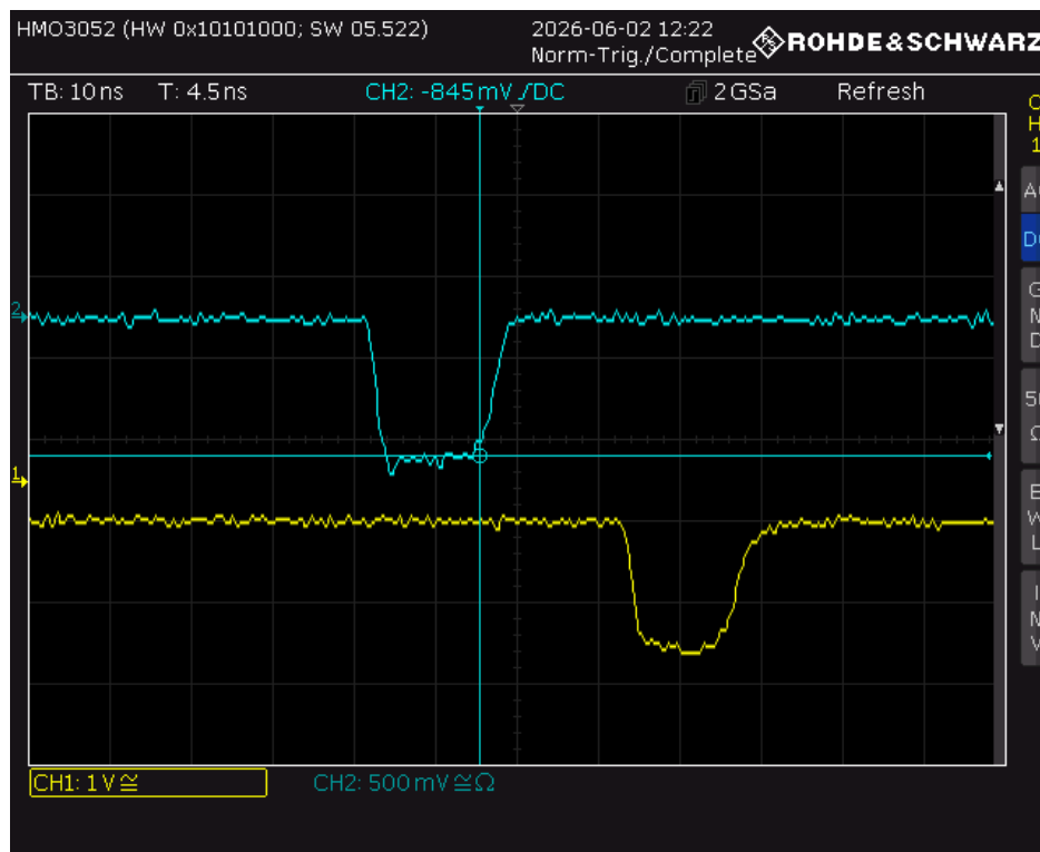
Abbildung 2.39: Oszillogramm des linken Fast-Signals über den CFD (CH 1) im Vergleich zu rechten Fast-Signal über CFD und ns-Delay (CH 2), wobei das ns-Delay auf 31.5 ns eingestellt ist. Die Signale sind nun zeitlich so ausgerichtet, dass sie innerhalb des Koinzidenzfensters liegen.
