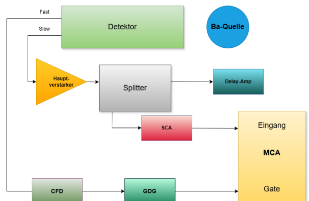
(b) Einstellung zur Aufnahme des Energiespektrums
