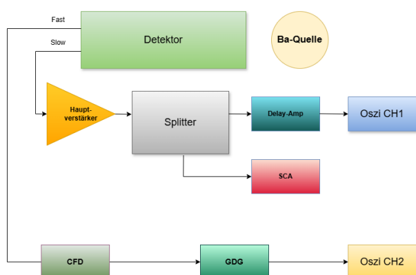
(a) Einstellung zur Herstellung der Koinzidenz zwischen Fast- und Slow-Signal
