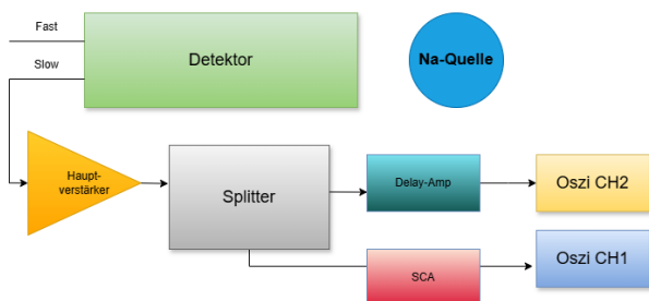
(a) Aufbau zur Untersuchung des SCA.
