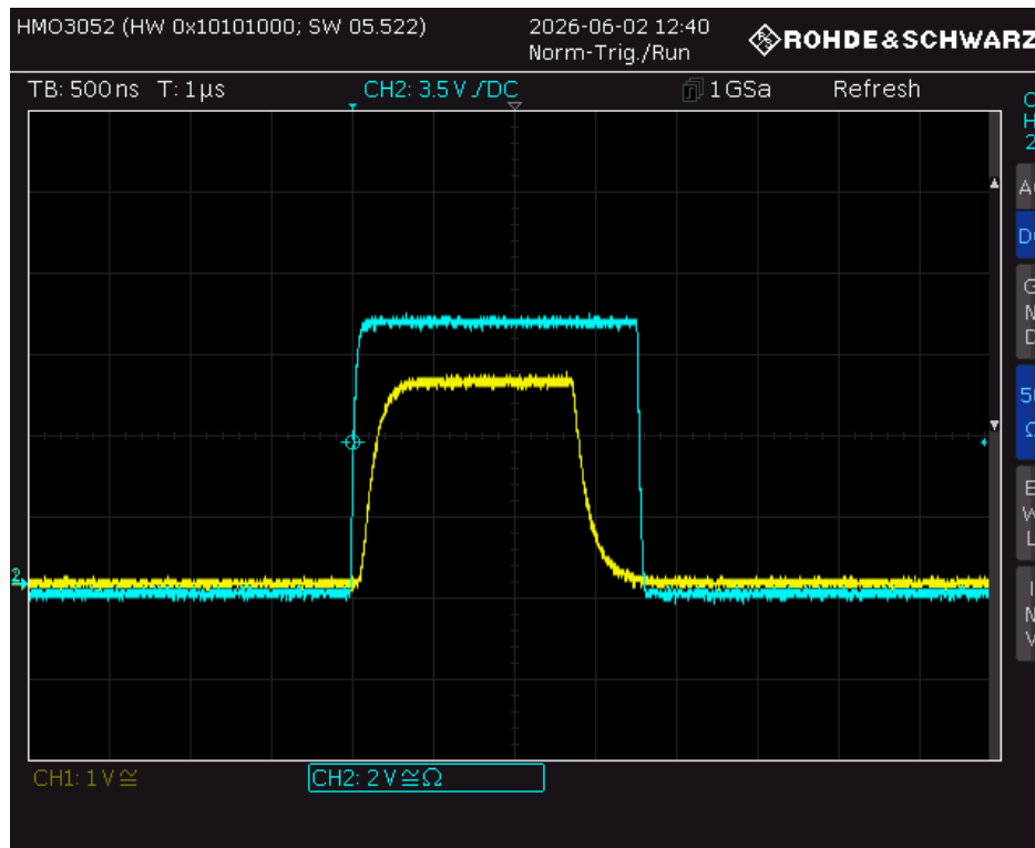
Abbildung 2.30: Oszillogramm vom TAC-Fastkreis (CH 1) und dem Slowkreis über Koinzidenzeinheit und GDG (CH 2)
