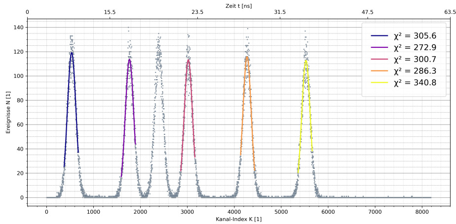
Abbildung 2.31: Messung der Promptkurve mit ^{22}\text{Na} am MCA
