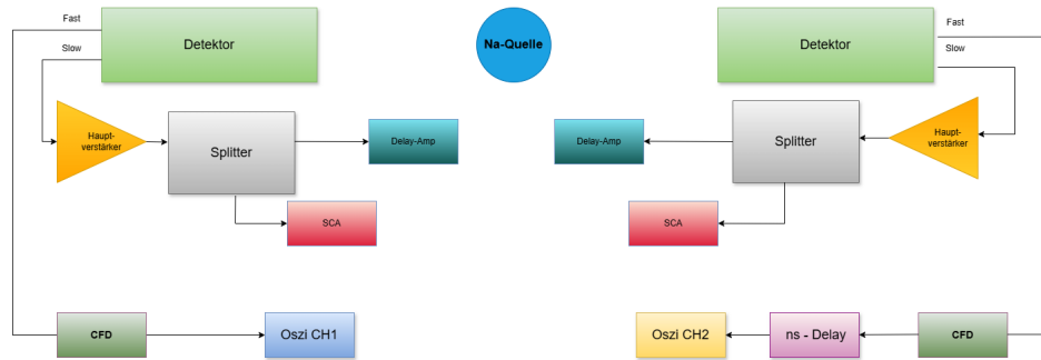
Abbildung 2.27: Schaltplan zur Einstellung der Verzögerung von Start- und Stopp-Signalen im Fast-Kreis.
