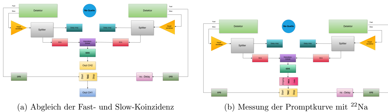
Abbildung 2.29: Schaltungspläne zum Abgleich der Fast- und Slow-Koinzidenzsignale sowie zur Aufnahme der Promptkurve mit ^{22}\text{Na} .
