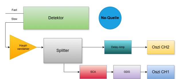
(b) Aufbau mit zusätzlichem Gate-Delay-Generator.
