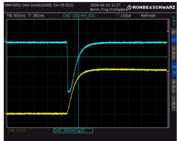
(b) Linker Detektor
