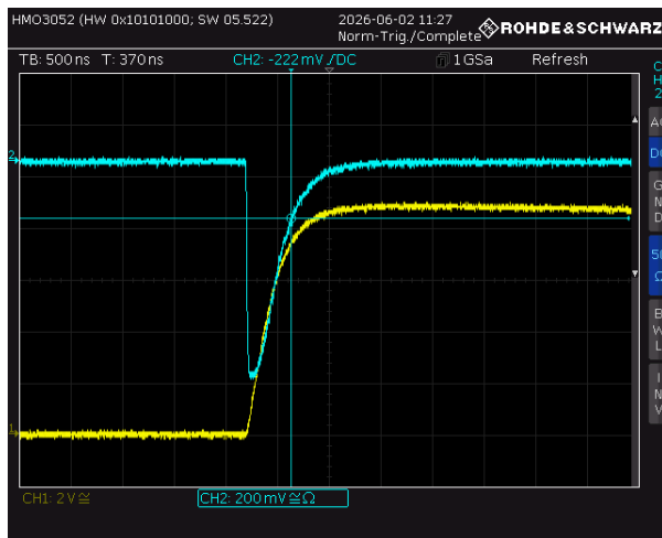
(a) Rechter Detektor
