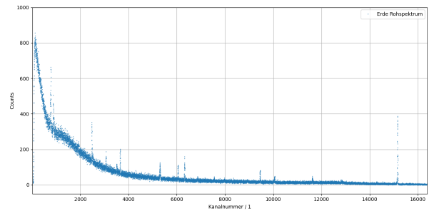
Abbildung 10.6: Am HPGe-Detektor gemessenes Langzeit-Spektrum mit der Bodenprobe.
