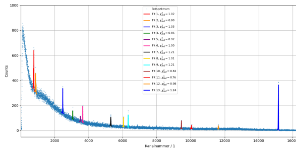
Abbildung 10.6: Am HPGe-Detektor gemessenes Langzeit-Spektrum mit der Bodenprobe.
