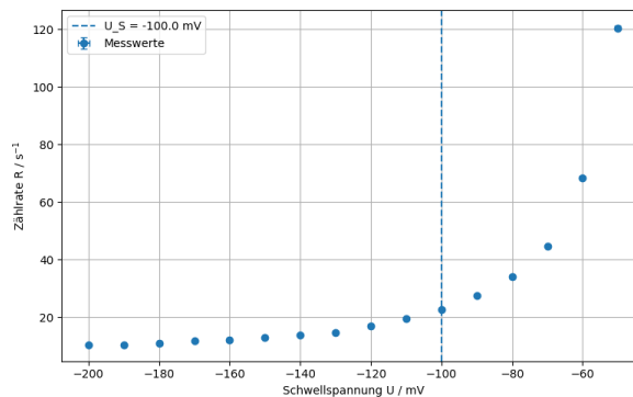
Abbildung 4.1: Schwellenkurve zur Bestimmung der Schwellenspannung vom Diskriminator D1
