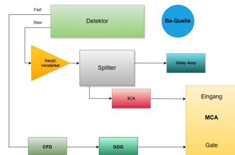
Abbildung 2.26: Mit dieser Einstellung wird das Energiespektrum aufgenommen.
