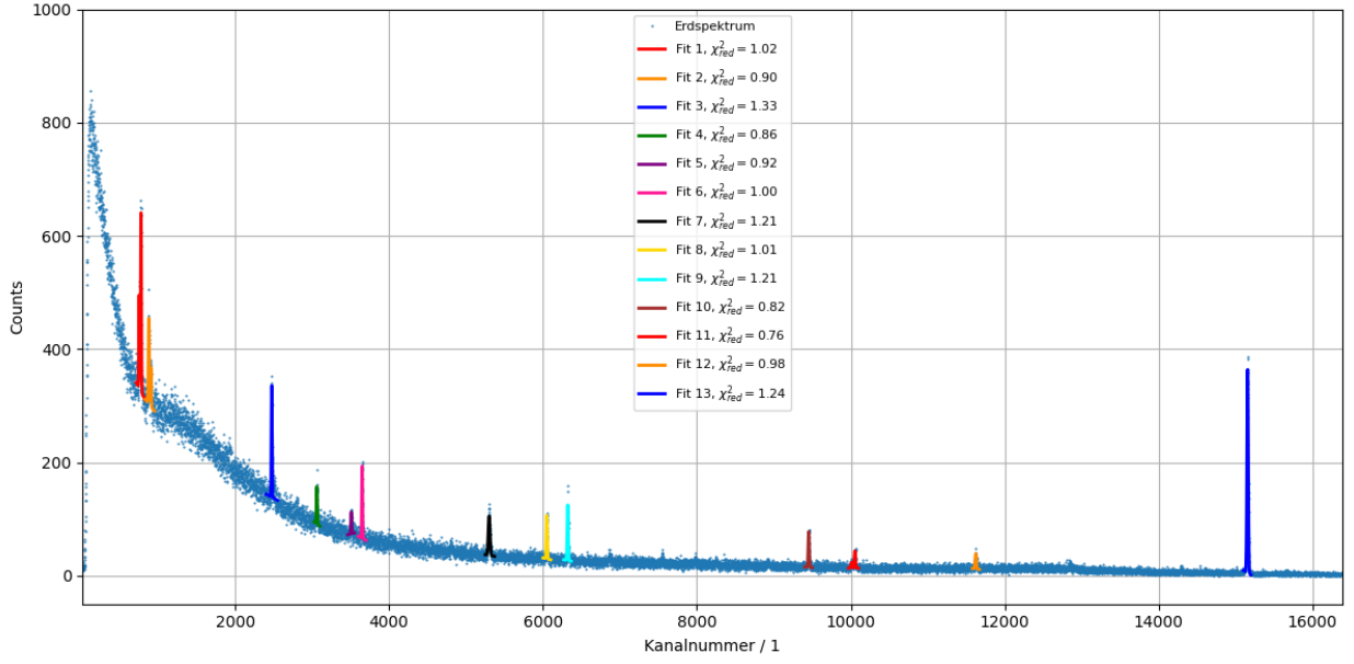
Abbildung 8.1: Gemessenes HPGe-Spektrum der untersuchten Blumenerdeprobe. Die eingezeichneten Kurven entsprechen den Gaußanpassungen der identifizierten Peaks. Eine Korrektur durch Subtraktion eines Hintergrundspektrums wurde nicht durchgeführt.
