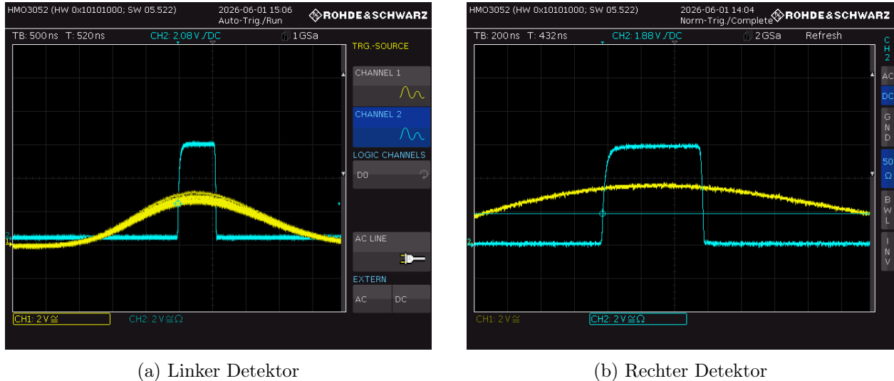
Abbildung 2.7: Oszillogramme des analogen Signals nach dem Delay-Verstärker (CH I) und des digitalen SCA-Signals (CH II) bei geöffnetem SCA-Fenster.
