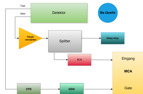
Abbildung 2.26: Mit dieser Einstellung wird das Energiespektrum aufgenommen.
