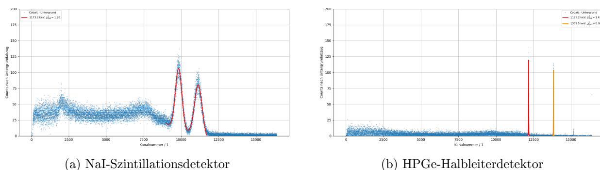
Abbildung 5.1: Gemessenes Energie-Spektrum der ^{60}\text{Co} -Quelle an beiden Detektoren
