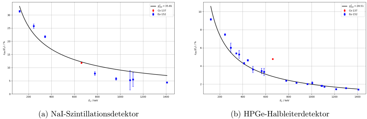
Abbildung 8.1: Effizienz \epsilon(E_\gamma) der Detektoren anhand des ^{152}\text{Eu} -Spektrums
