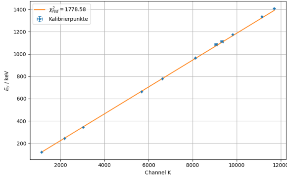
(a) NaI-Szintillationsdetektor
