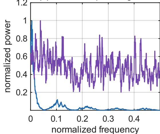
(d) Smoothed periodograms
