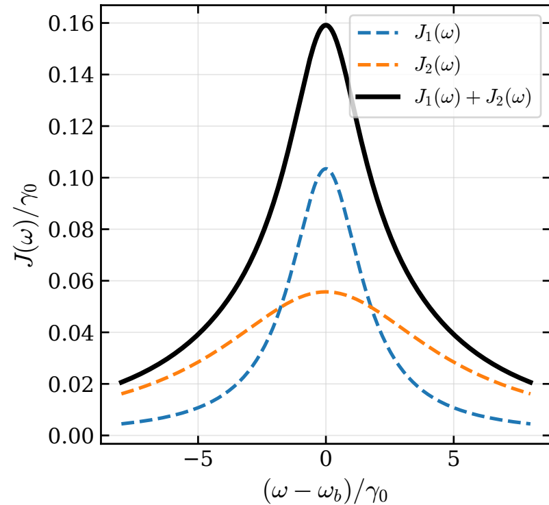
Bi-Lorentzian spectrum
