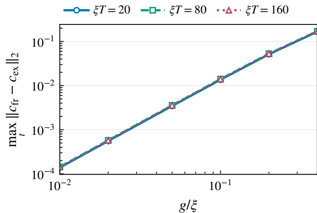
(d) Frozen-memory approximation
