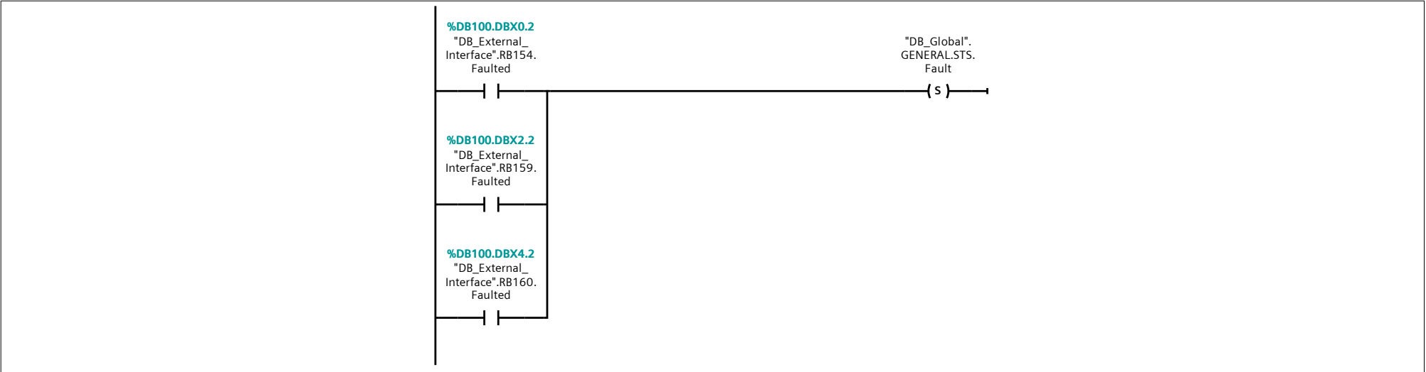
Network 4: Luces de indicaciones segun la condicion de la instalacion.
