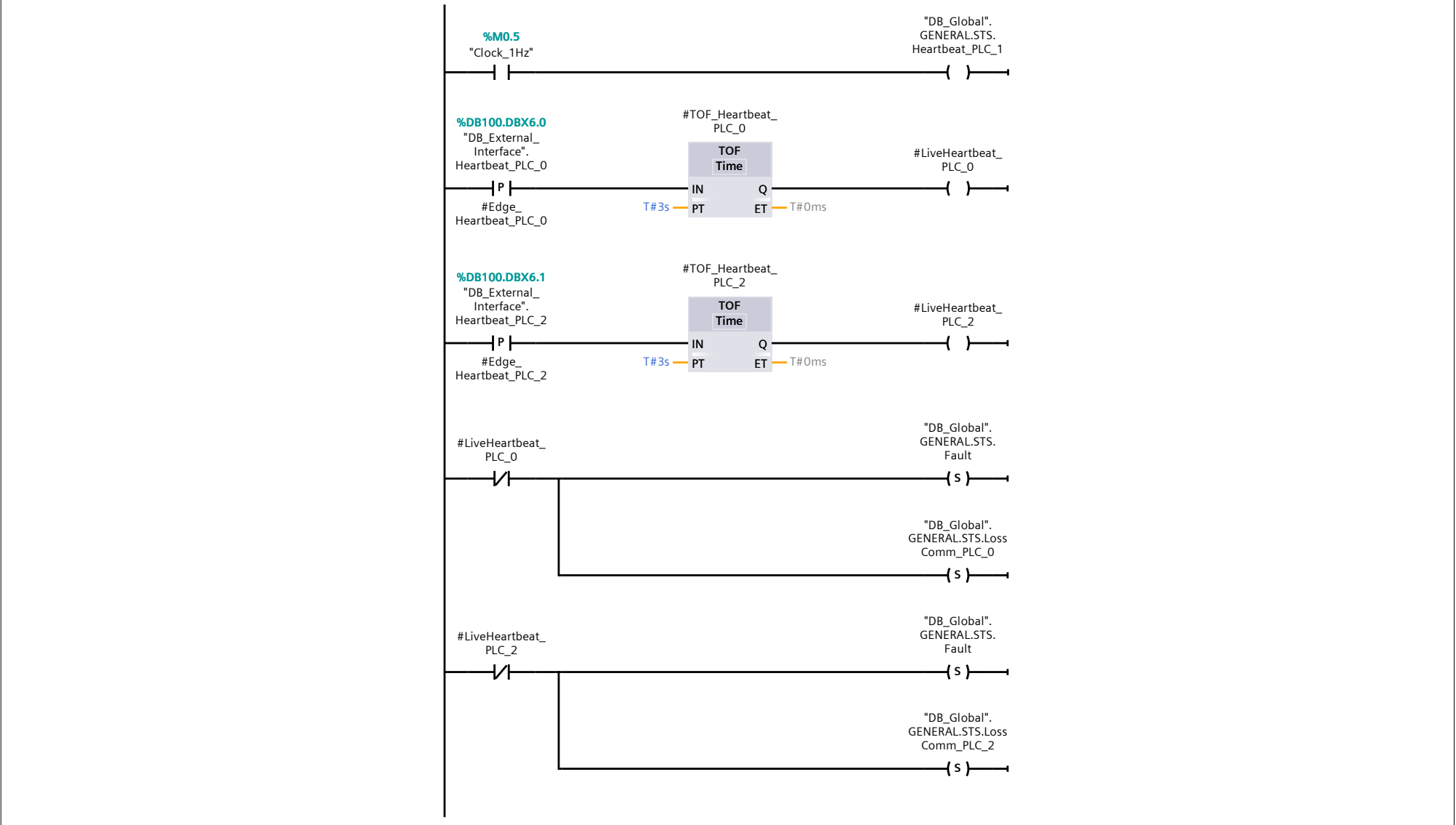
Network 3: Verificacion de fault en RB precedentes y proximas
