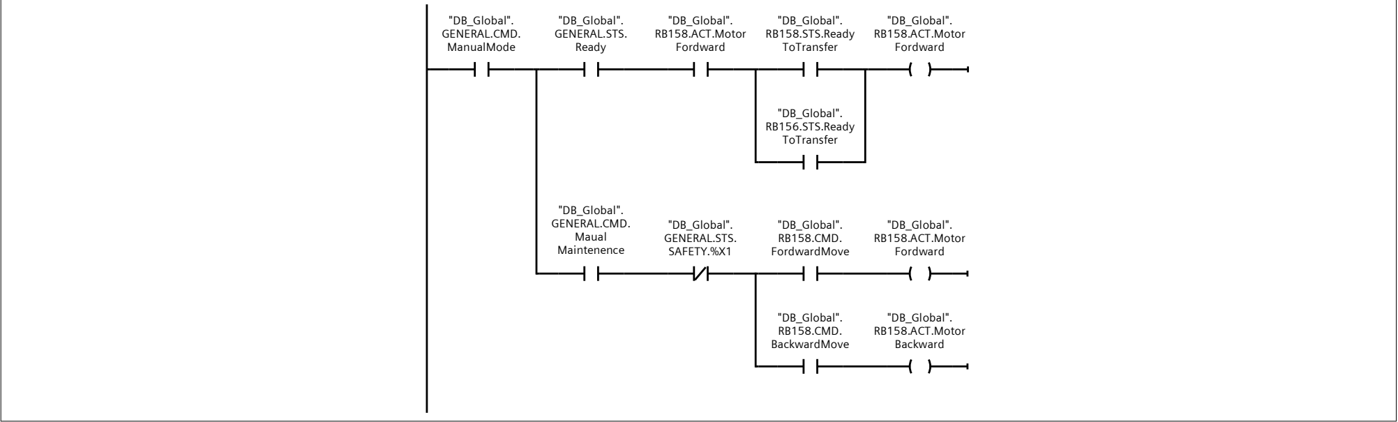
Network 5: Validacion de condiciones para hacer set de transferencia en manual
