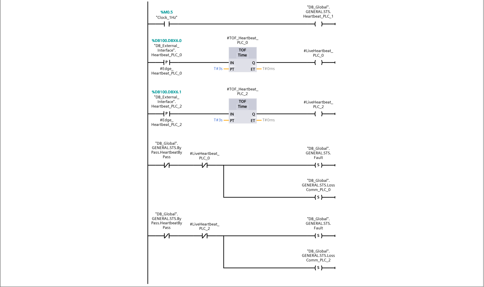
Network 3: Verificacion de fault en RB precedentes y proximas
