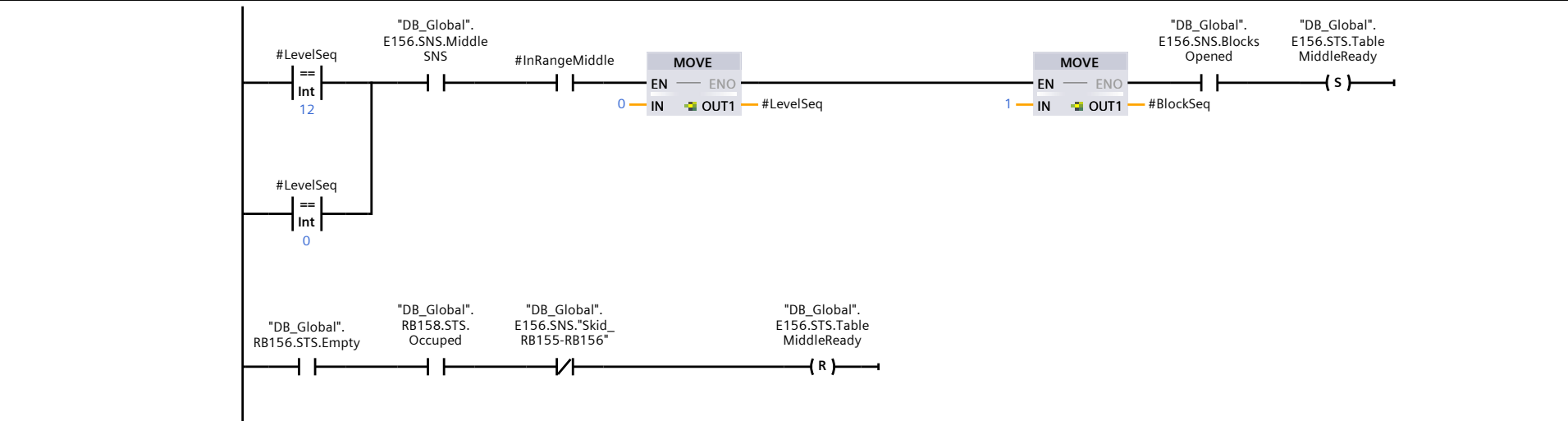
Network 7: mandar al comando a bajar a nivel bajo
