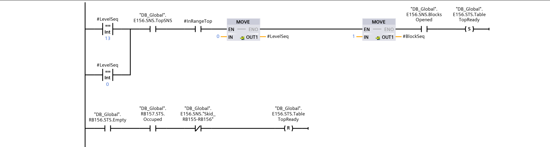
Network 9: validacion para bajar el ascensor de nivel bajo
