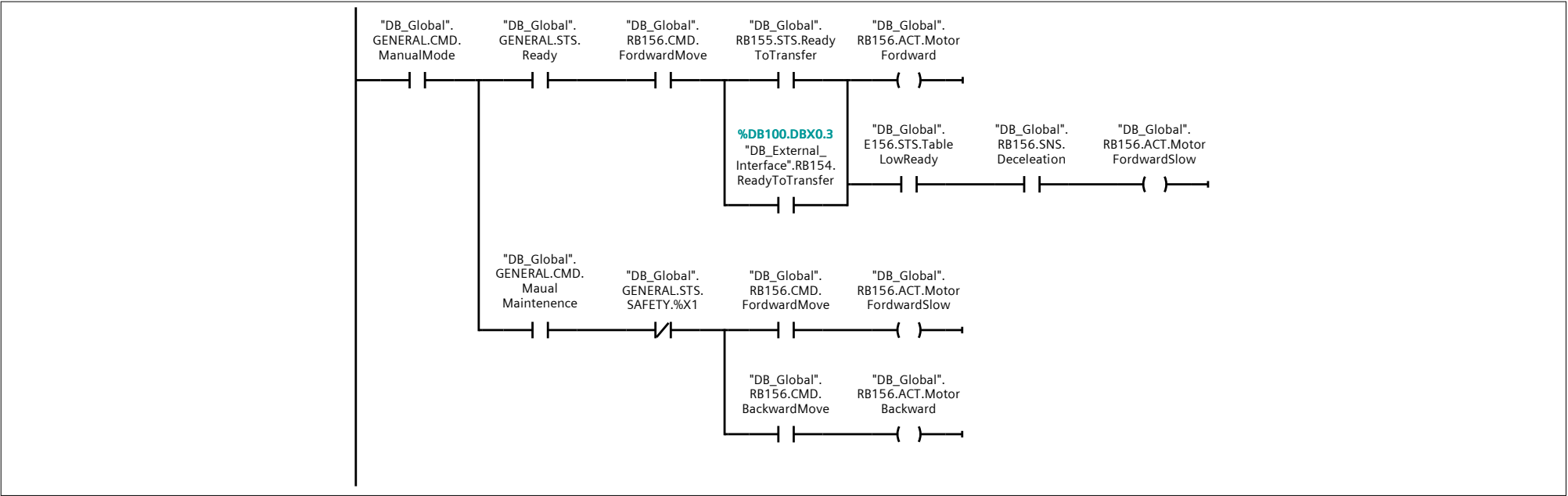
Network 6: Validacion de condiciones para hacer un set de transferencia en manual
