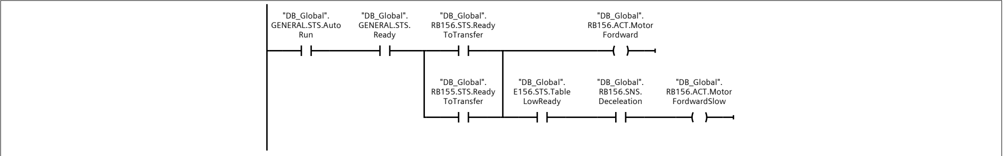
Network 5: Determinacion de movimientos en manual
