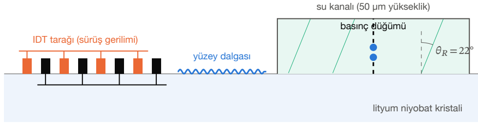
Şekil 3: Cihazın kesiti. Tarak biçimli bir elektrot kristal yüzeyi boyunca bir dalgalanma sürer. Dalgalanma kristalde (3979 m/s) sesin suda gittiğinden (1497 m/s) daha hızlı gittiği için, sıvıya sabit bir açıyla, yaklaşık 22^\circ ile sızar — bir bardak sudaki pipetin kırık görünmesiyle aynı nedenle. Karşılıklı iki yönden gönderilen iki böyle dalga duran örüntüyü oluşturur.
