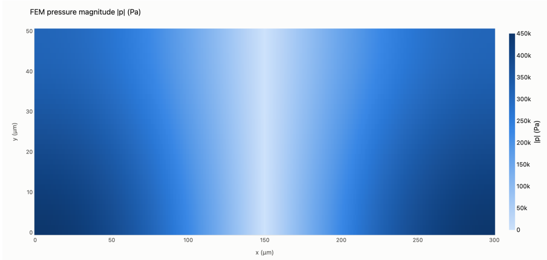
Şekil 9: Kanal kesitinde hesaplanan basınç alanı. Koyu mavi basıncın en sert salındığı yer; ortadaki soluk dikey şerit ise hiç değişmediği düğüm — hücrelerin toplandığı yer. Kanal 300 \mu\text{m} geniş, 50 \mu\text{m} yüksektir. Koyu bantların yukarı doğru soluklaştığına dikkat edin: ses tavandan sızıp gider ve bu soluklaşmanın çok önemi vardır (§27).
