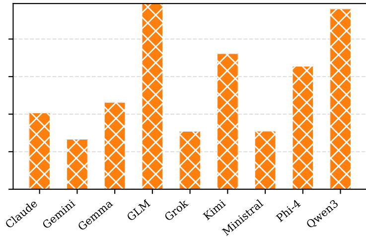
llm-iac
