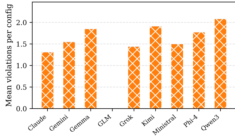
IaC-Eval
