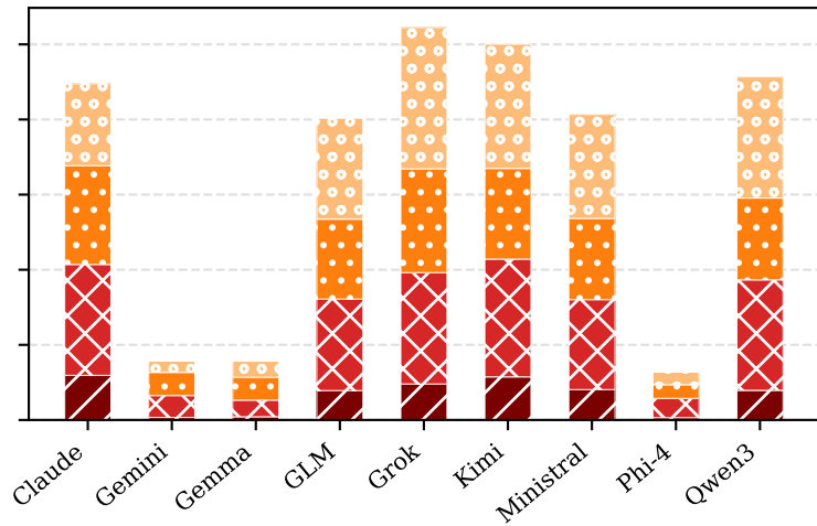
llm-iac
