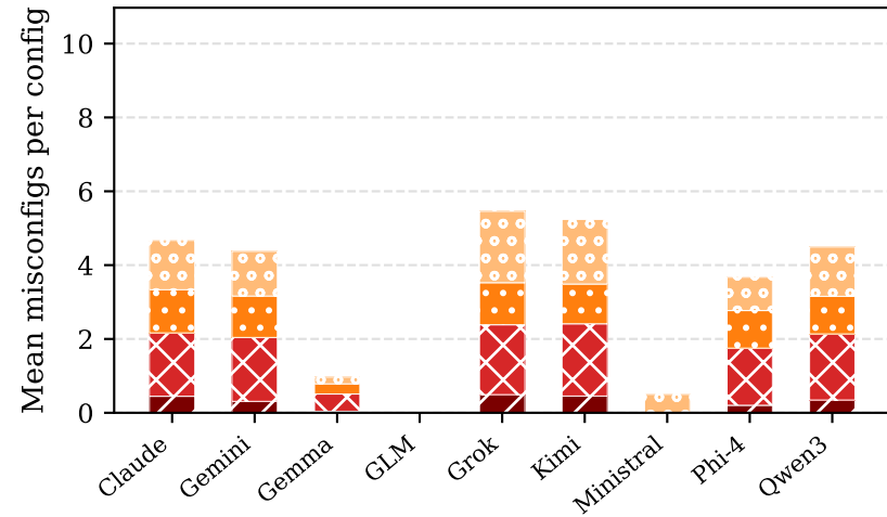
IaC-Eval
