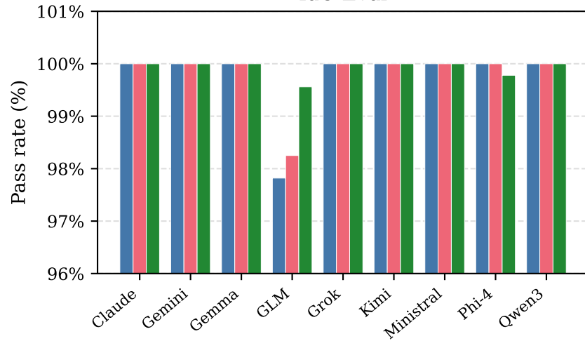
IaC-Eval
