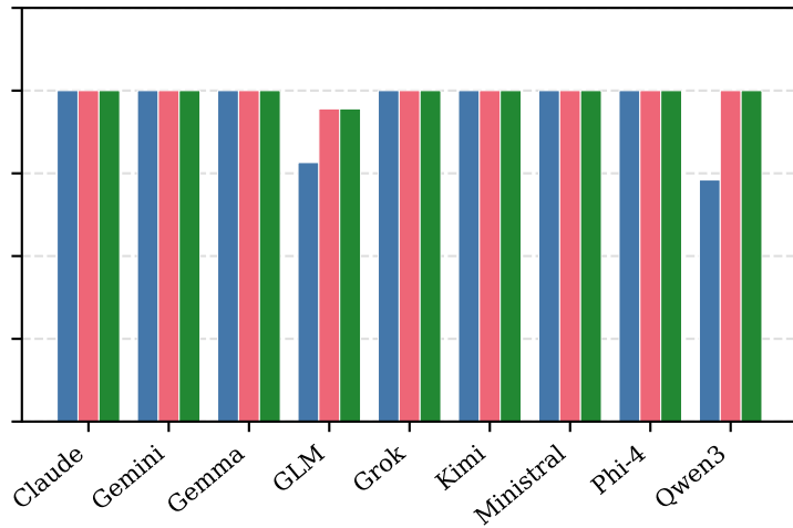
llm-iac
