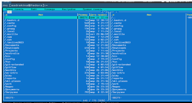
Рис. 2: Запуск команды.
