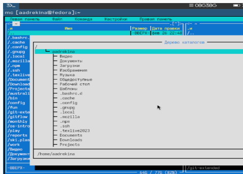
Рис. 7: Дерево каталогов.
