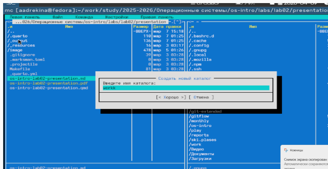
Рис. 3: Создание каталога.
