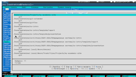
Рис. 5: Поиск файлов.
