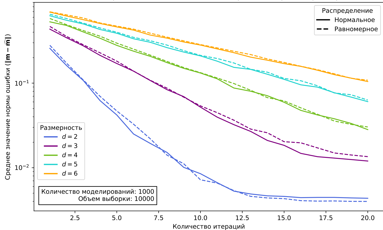
Зависимость нормы ошибки от количества итераций для разных размерностей
