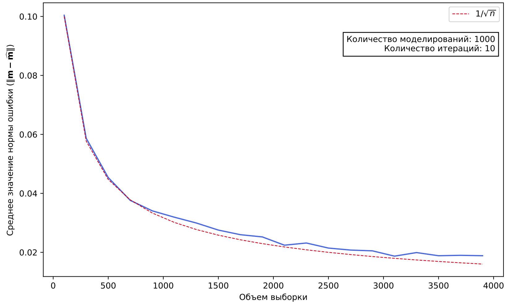
Зависимость нормы ошибки от объема выборки
