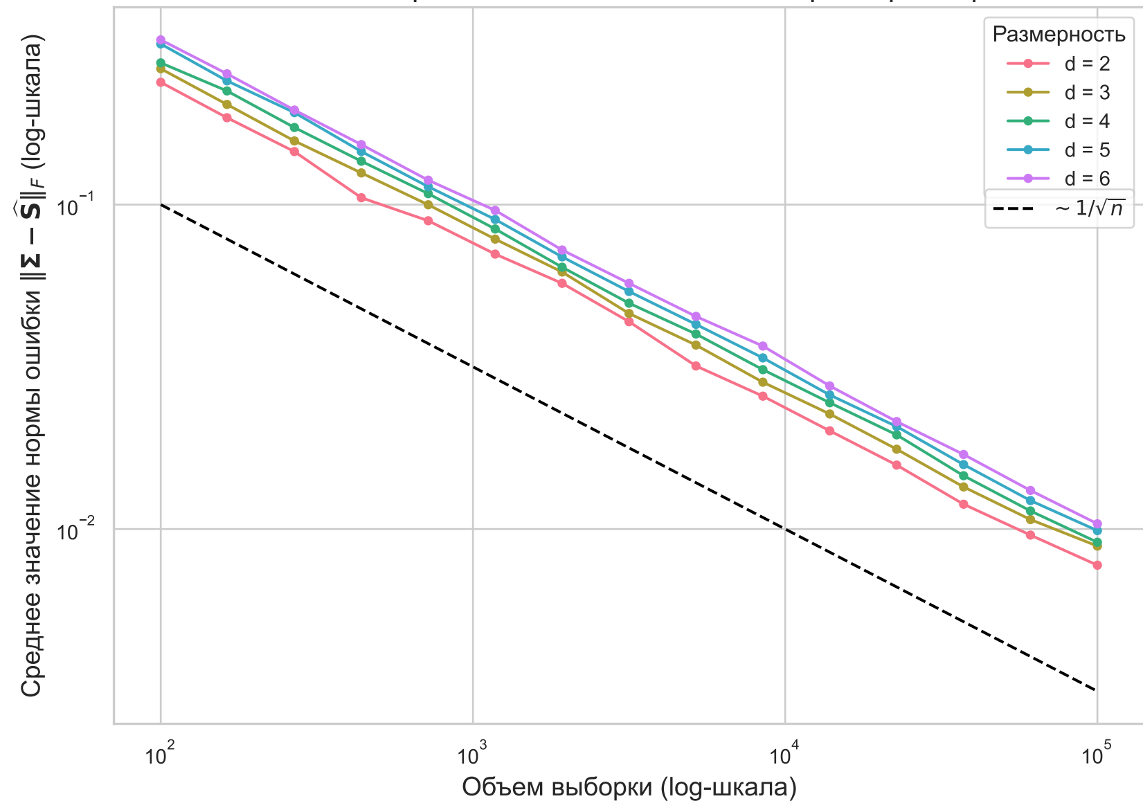
Зависимость нормы ошибки от объема выборки и размерности
