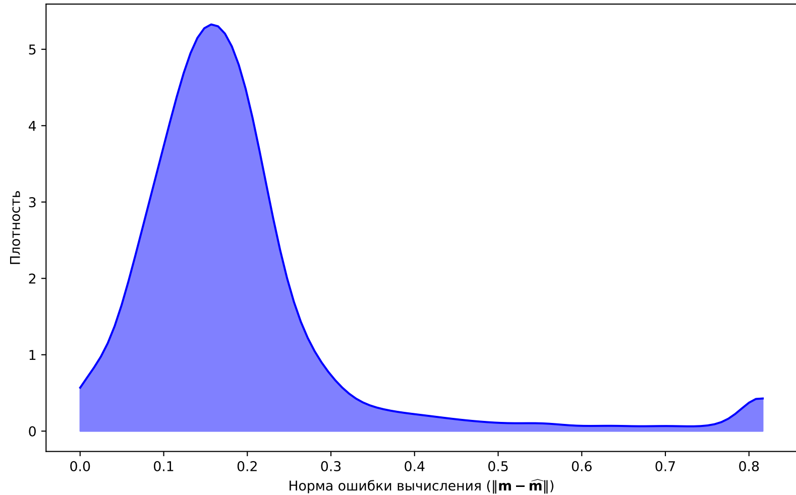
Оценка плотности вероятности ошибки
