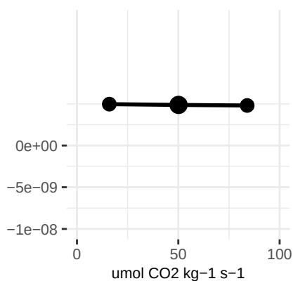
SLA
