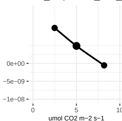
AmaxFrac
