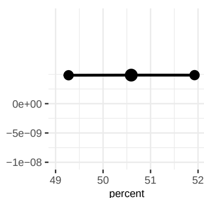
stem_respiration_rate
