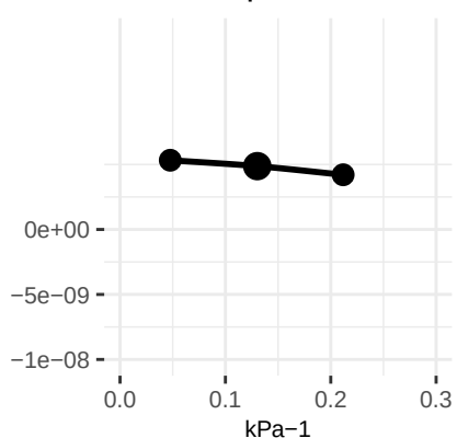
coarse_root_respiration_Q10
