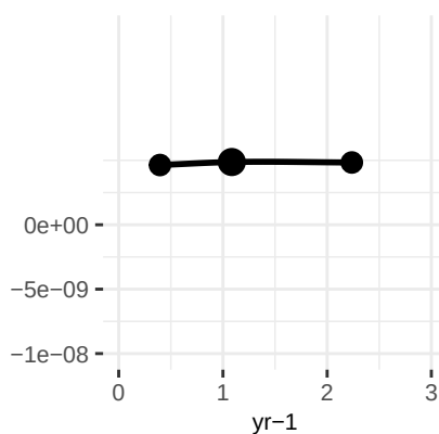
leaf_respiration_rate_m
