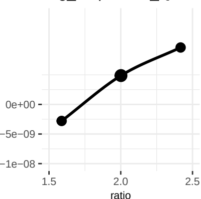
veg_respiration_Q10
