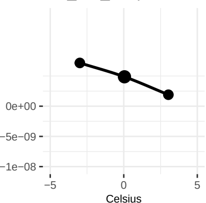
extinction_coefficient
