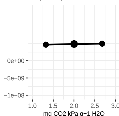
dVpdExp
