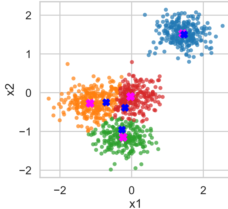
DP-GRAMS-C
