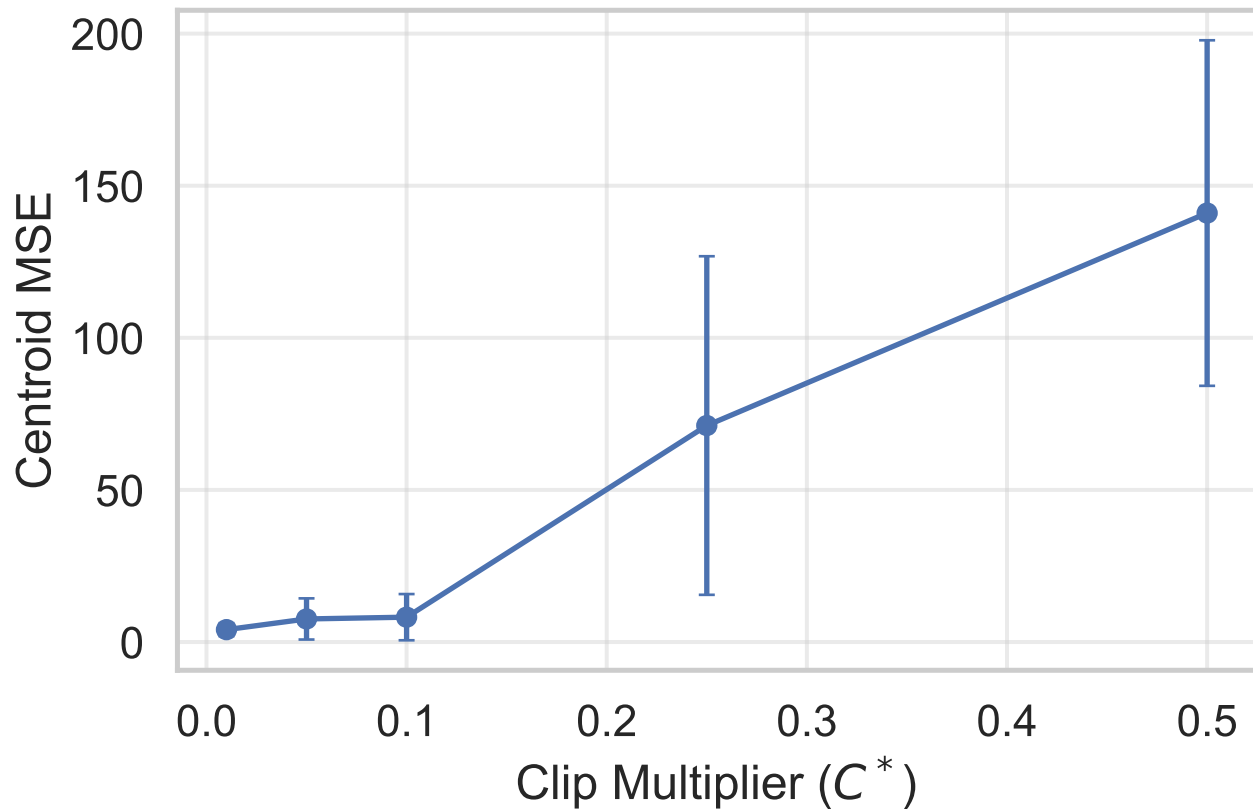
DP-GRAMS-C on Iris: MSE vs C^*
