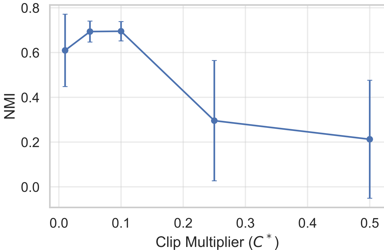
DP-GRAMS-C on Iris: NMI vs C^*
