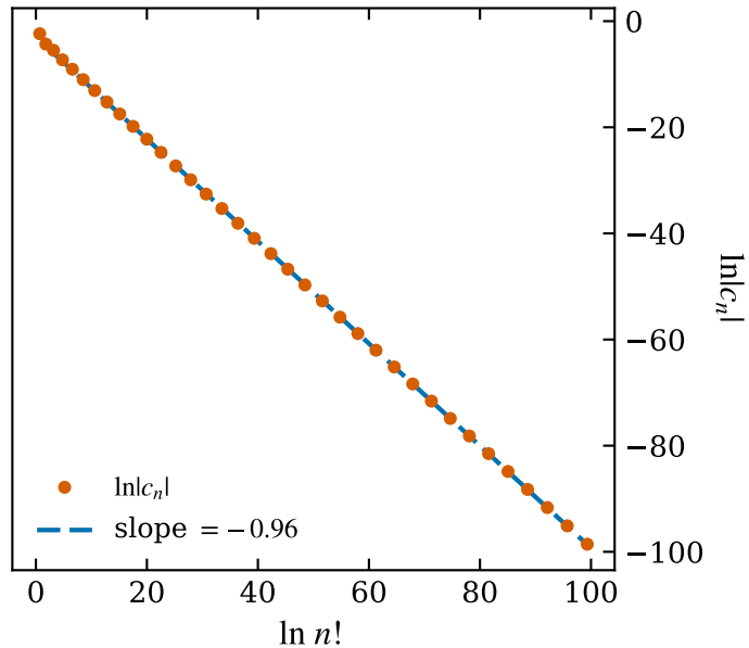
|c_n| \sim (n!)^{-0.96} : super-exponential
