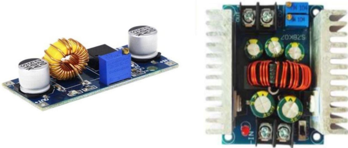
Şekil 6: XL4015 DC-DC voltaj düşürücü (Direnc.net. 2026) ve SZBK07 DC-DC voltaj düşürücü (XLSEMI. 2026).
