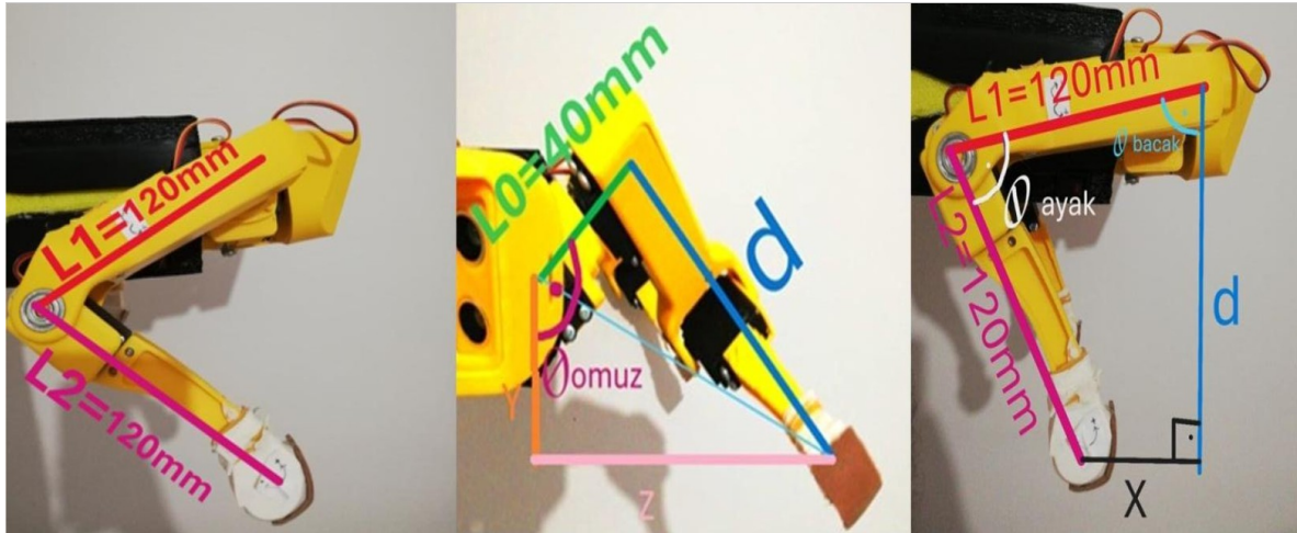
Şekil 13: Kinematik hesaplamalar ve bacak segman uzunlukları.
