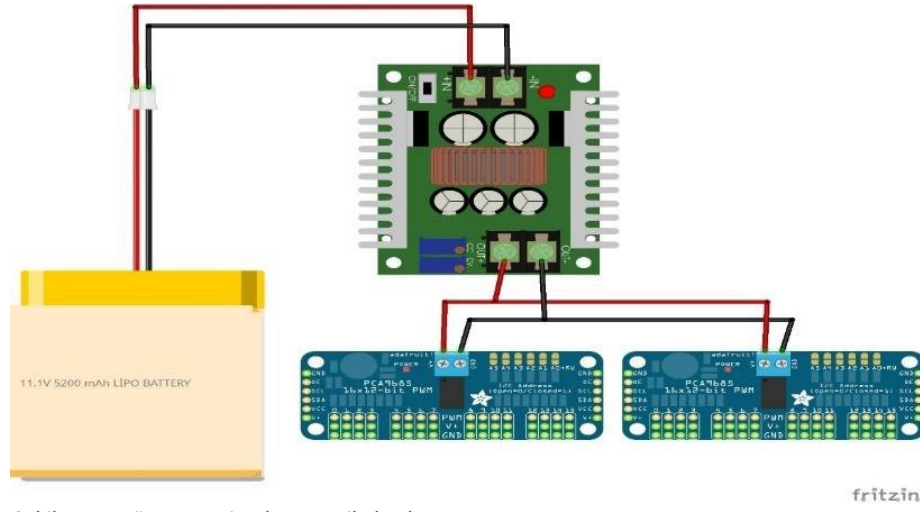
Şekil 11: 5. yöntem – LiPo batarya ile besleme.
