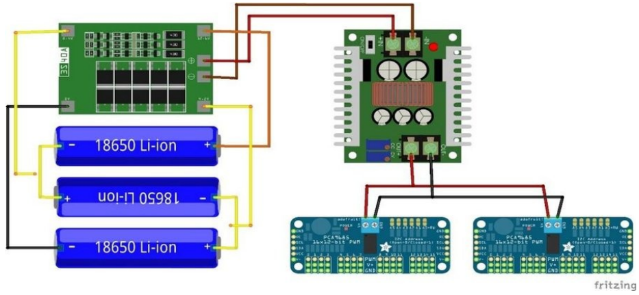
Şekil 9: 3. yöntem – sürücü kartı ayırımı.
