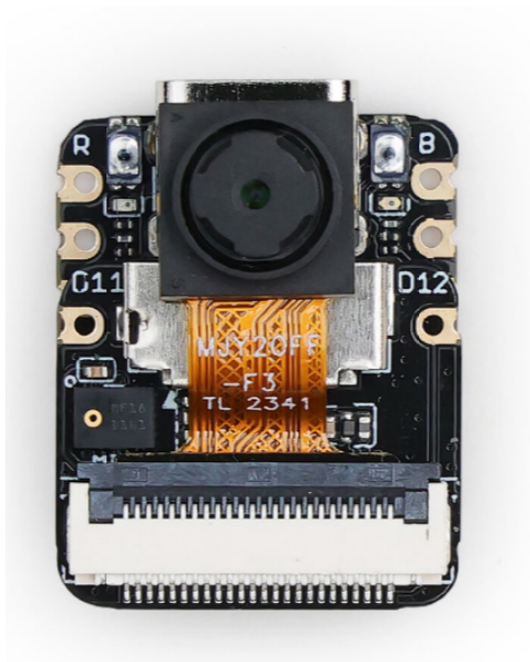
Figura 2.16: XIAO ESP32 CAM Fuente: Adaptado de [12]
