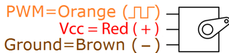
Figura 2.26: Distribución de cables Fuente: Adaptado de [36]
