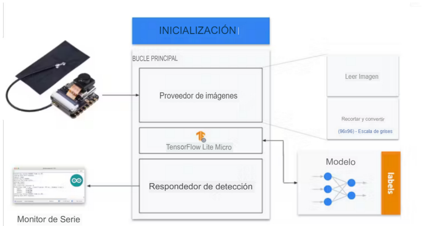
Figura 3.1: ESP32 CAM y Machine Learning Fuente: Adaptado de [43]
