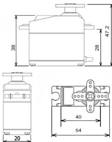
Figura 2.25: Dimensiones del servo motor Fuente: Adaptado de [36]
