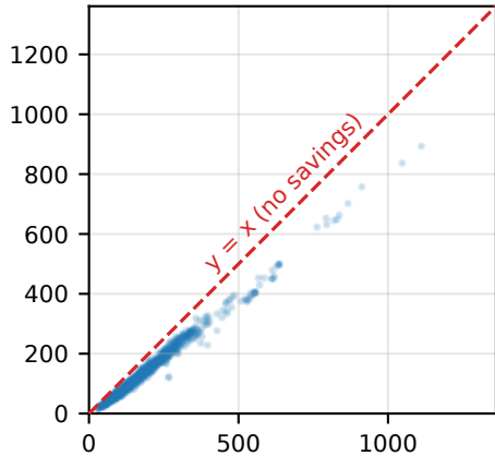
tiktoken (o200k_base)
