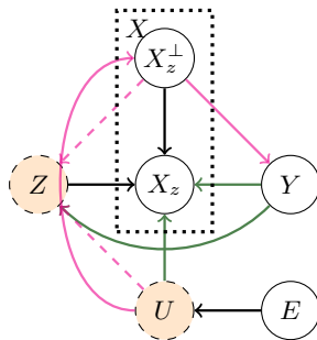
(b) \mathcal{G}_2 : confounded-descendant
